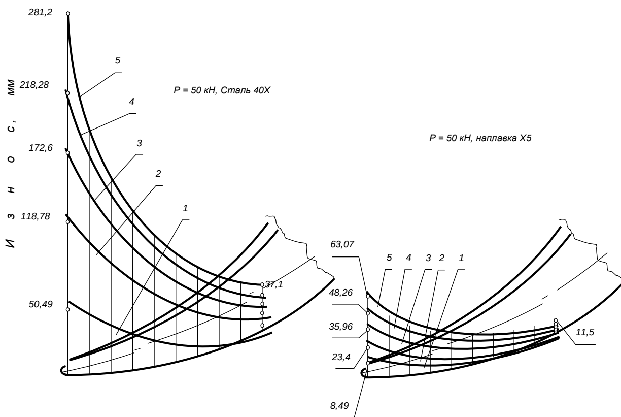
Изменение формы режущей части биомеханической модели в процессе изнашивания при наработке: 1- 120 час; 2- 360 час.; 3-600 час.; 4- 840 час.; 5- 1200 час.
