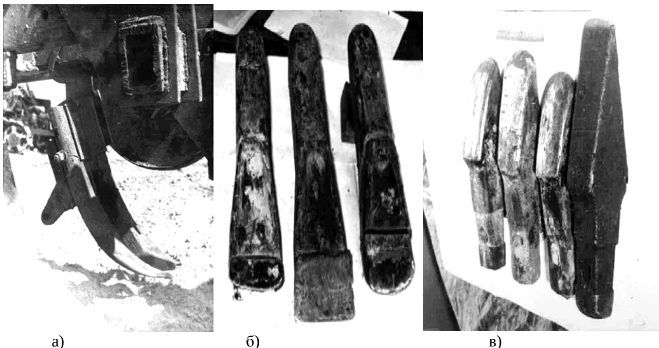
а) Общий вид рабочего органа рыхлителя на базе бульдозера ДЗ-42 Общий вид клиновидных зубьев ковшей экскаваторов ЭО –4121 (б) и ЭО – 3322 (в)
