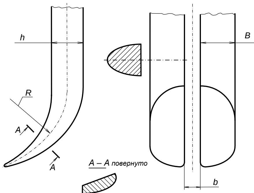
Конструктивная схема лабораторных образцов биологического прототипа криволинейных моделей
