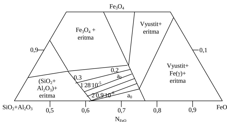
8.11-rasm. 1200°C da \text{FeO}-\text{Fe}_2\text{O}_3 (\text{Fe}_3\text{O}_4) - \text{SiO}_2 sistemada komponentlarni aktivlik diagrammasi.
