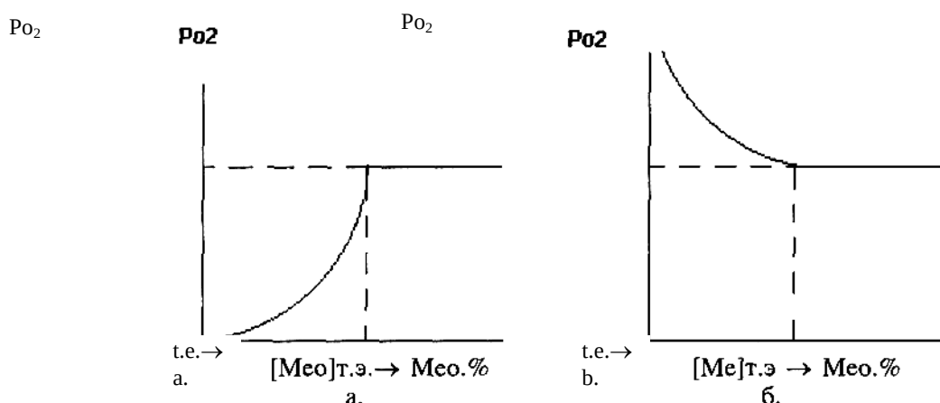
3.1- rasm. Oksid ajralish tarangligining MeO ni shlakdagi (a) va Me ni eritmada (b) miqdoriga bog‘liqligi.
