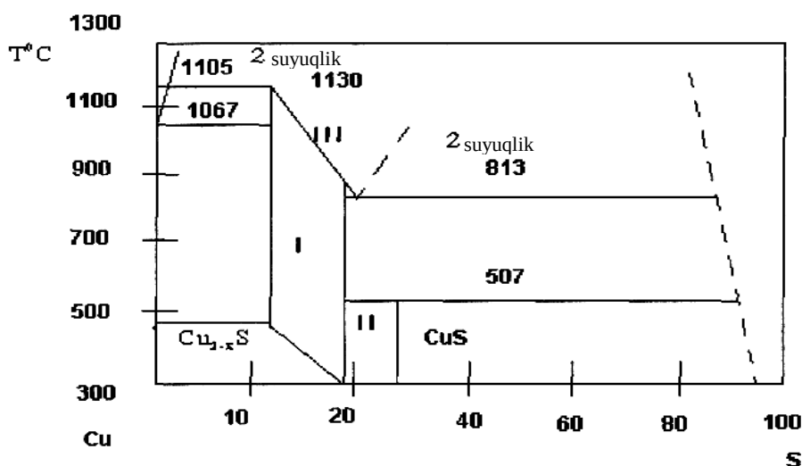
2.3-rasm. Cu-S sistemaning muvozanat diagrammasi.
