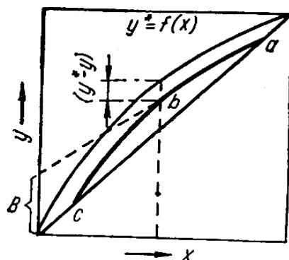
12.5-rasm. Rektifikatsion kolonnani muvozanat va ishchi chiziqlari.
