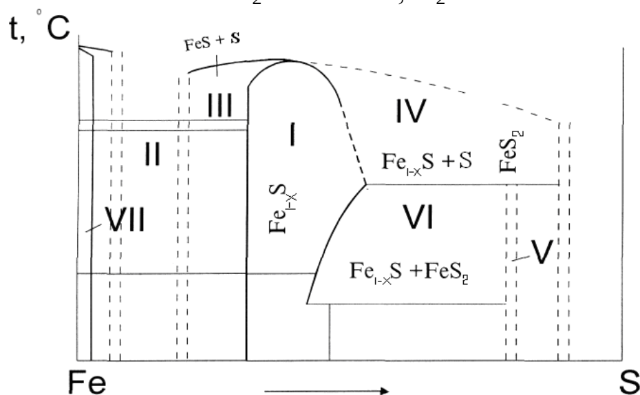
2.6- rasm. Fe-S sistemasining holat diagrammasi.
