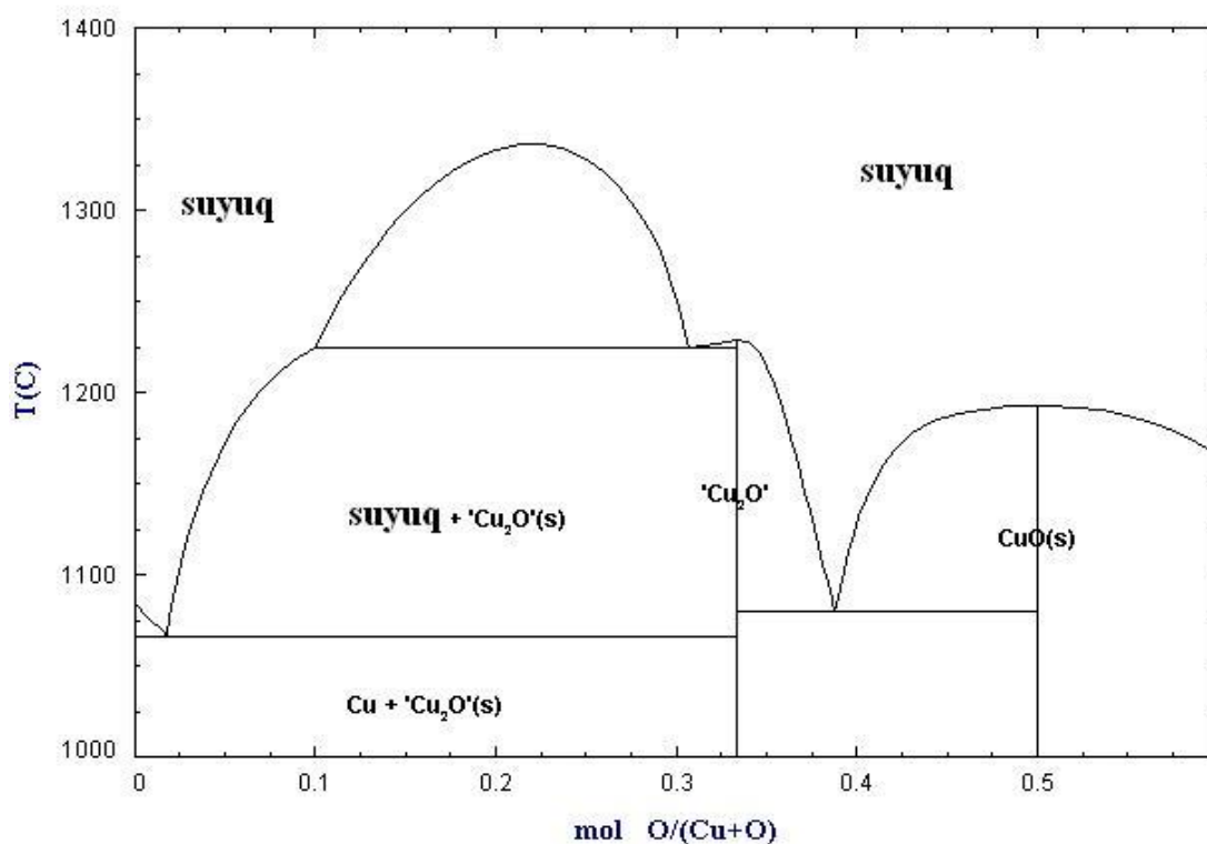
2.5-rasm. Cu – O sistemasining holat diagrammasi.
