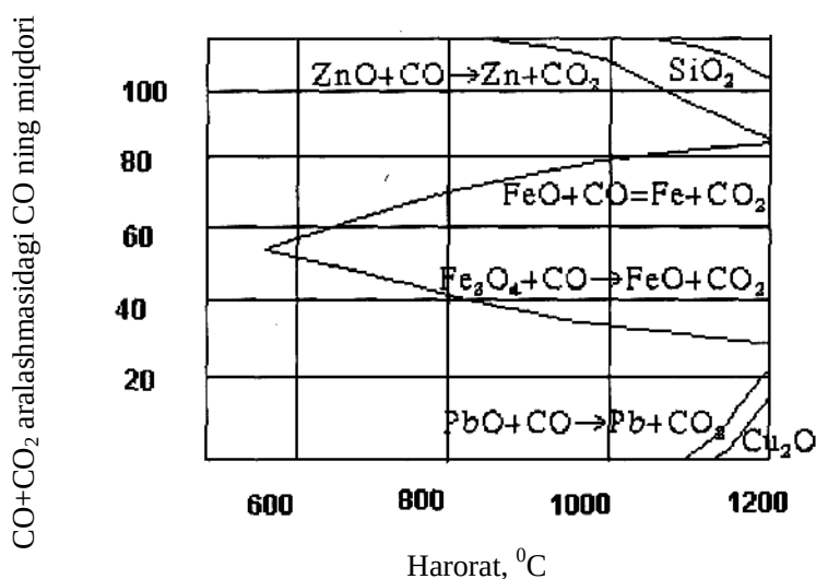
6.1-rasm. CO bilan oksidlarni tiklanish reaksiyasini muvozanatli gaz tarkiblari.
