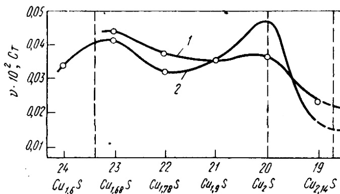
8.9-rasm. Cu - S sistemasini yopishqoqlik izotermasi.
