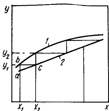
12.6-rasm. Rektifikatsion kolonnani nazariy likopchalar sonini aniqlash.
