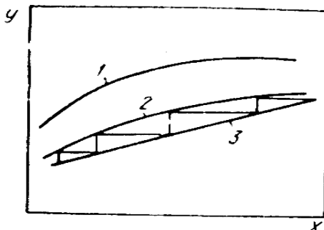
12.7-rasm. Rektifikatsion kolonnaning haqiqiy likopchalarning sonini aniqlash:
