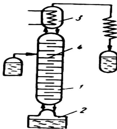
12.3-rasm. Rektifikatsion dastgohning sxemasi. 1-kolonna; 2- kub; 3- deflikmator; 4-ta'minlovchi likopcha.
