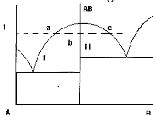
2.2- rasm. Bitta kimyoviy birikmali sistemaning holat diagrammasi.
