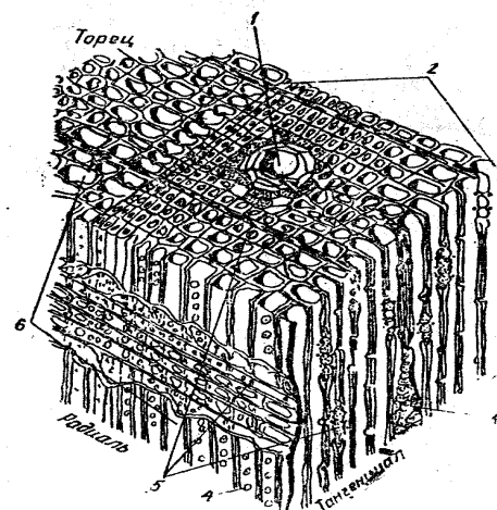
31-rasm. Qarag'ayning mikrostrukturasi.
