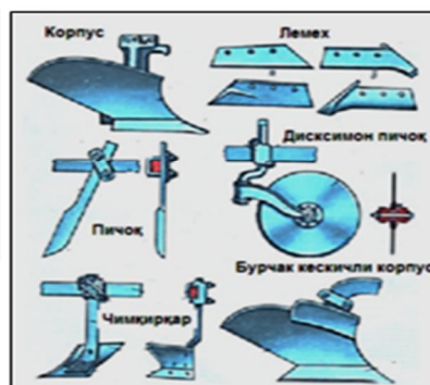
Плугнинг асосий қисмлари ва уларни ростлаш ўлчамлари: 1-рама; 2-чимқарқар; 3-дискли пичок; 4-асосий ағдаргич (корпус)
