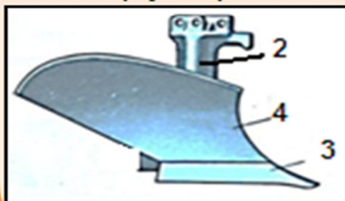
1-чимқарқар; 2-корпус; 3-лемех; 4-ағдаргич
