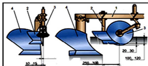
Плугнинг асосий қисмлари ва уларни ростлаш ўлчамлари: 1-рама; 2-чимқарқар; 3-дискли пичок; 4-асосий ағдаргич (корпус)
