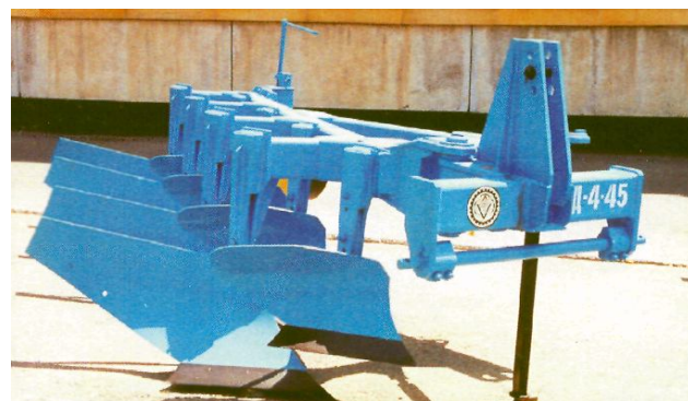
1.13-rasm. PD-4-45 ikki yarusli to'rt korpusli osma plug, sho'rlanmagan toshsiz yerlarni 40 sm gacha chukurlikda haydashga mo'ljallangan
