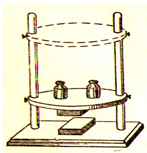
7.1-расм. Тупроқ қовушқоқлигини аниқлайдиган Аtterберг асбоби
