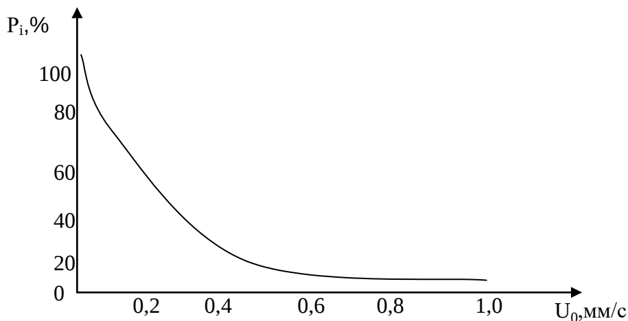
1-rasm. Choʻkmaga kelib tushgan muallaq zarrachalar miqdori ( P_i ) ning gidravlik yirikligi ( U_0 ) ga bogʻliqligi.
