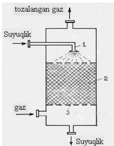
Absorberning sxemasi.
