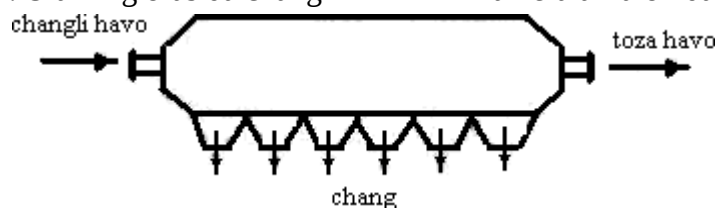
1-rasm. Gorizonta chang cho'ktirish kamerasi.
