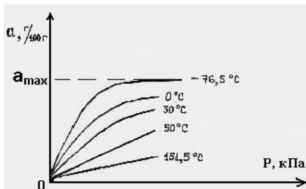
12-rasm. Faollashtirilgan ko'mirga uglerod qo'sh oksidi ( \text{SO}_2 ) adsorbsiyanish izotermalari.
