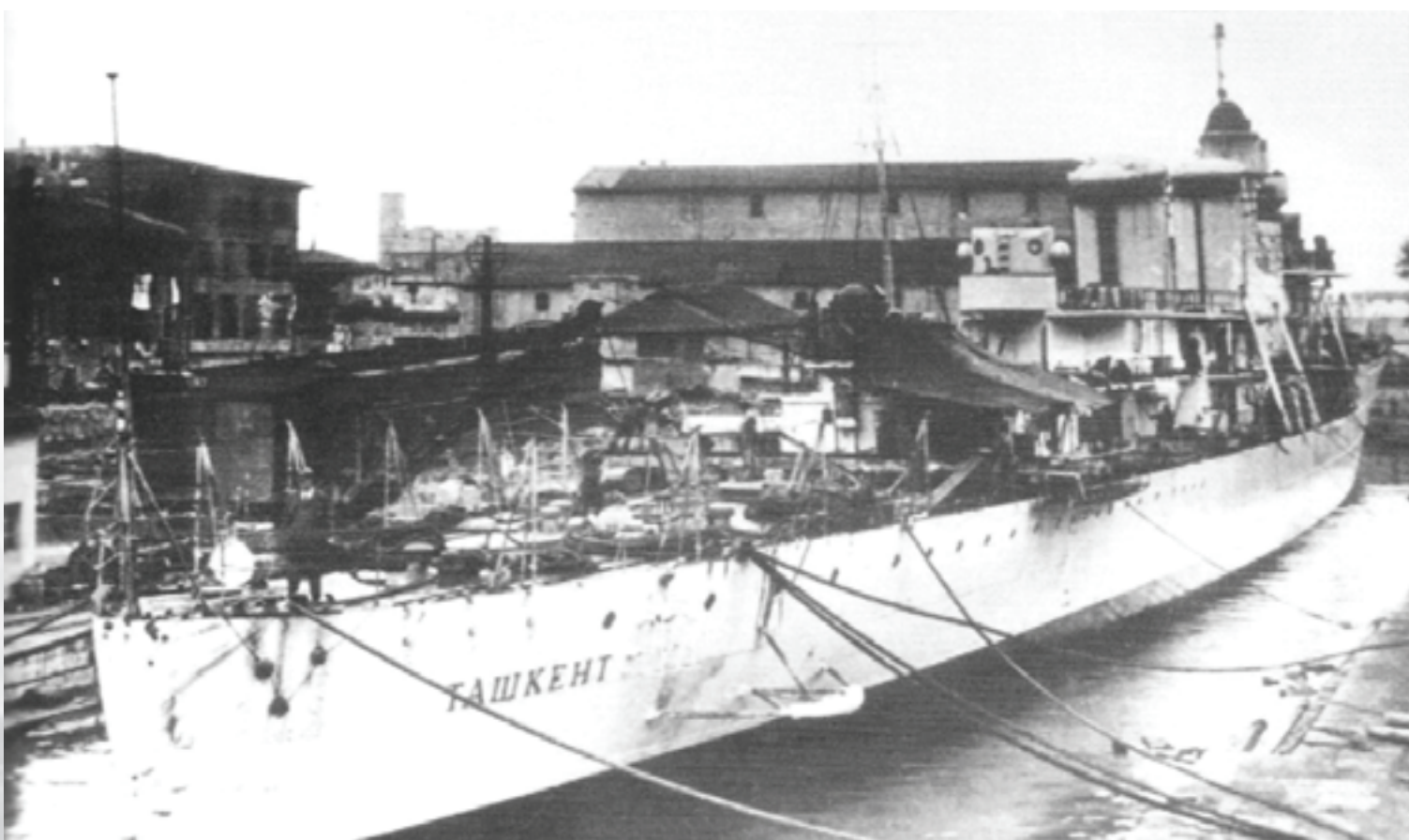
Лидер “Тошкент” Италиянинг “О.Т.О” фирмасининг Ливорнодаги корхонасида (тўлиқ қуриб битказилган ҳолати)
