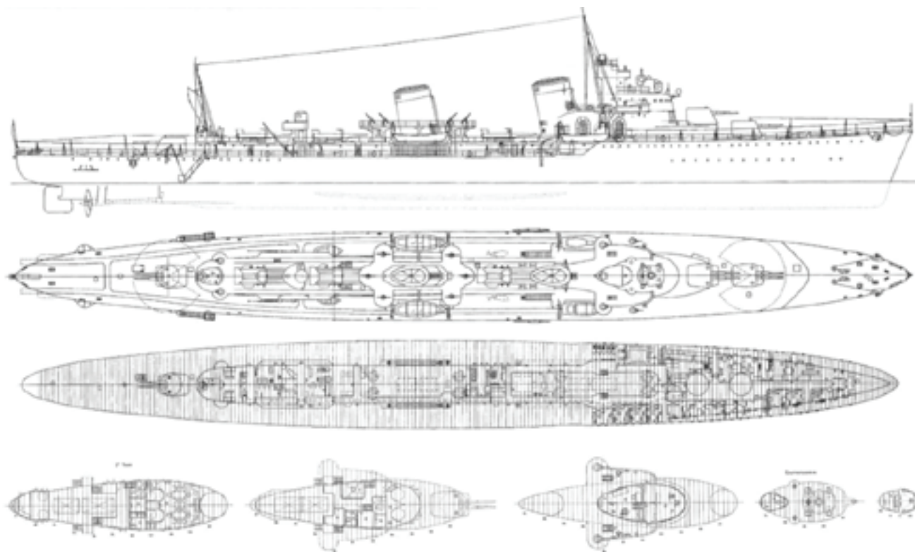
Италиянинг “О.Т.О” фирмаси томонидан тайёрланган Лидер “Тошкент”нинг ташқи чизмаси
