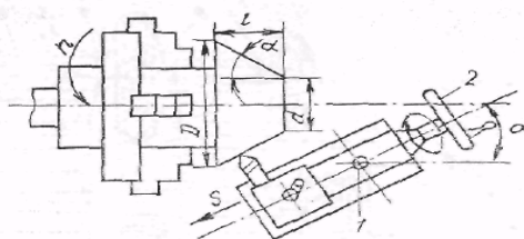
71-рasm. Суппорт устки салазаксини бурши би- лан конусавий юзларни йўниш: 1 — устки салазка; 2 — даста.
