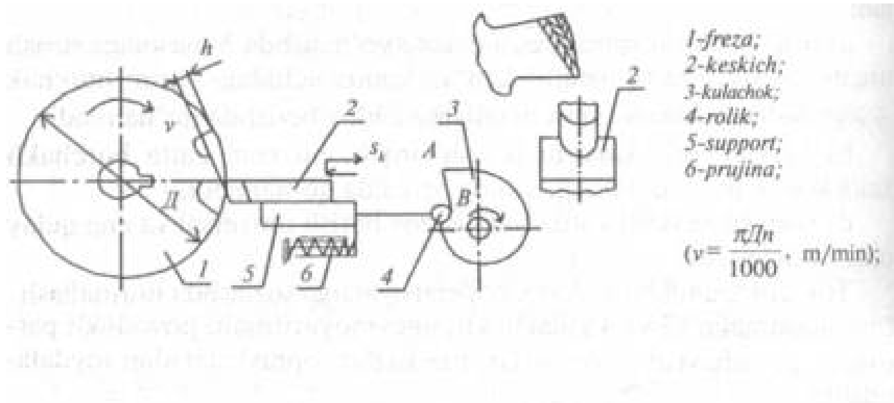
1-rasm. Freza orqa yuzasini gardanlash sxemasi.
