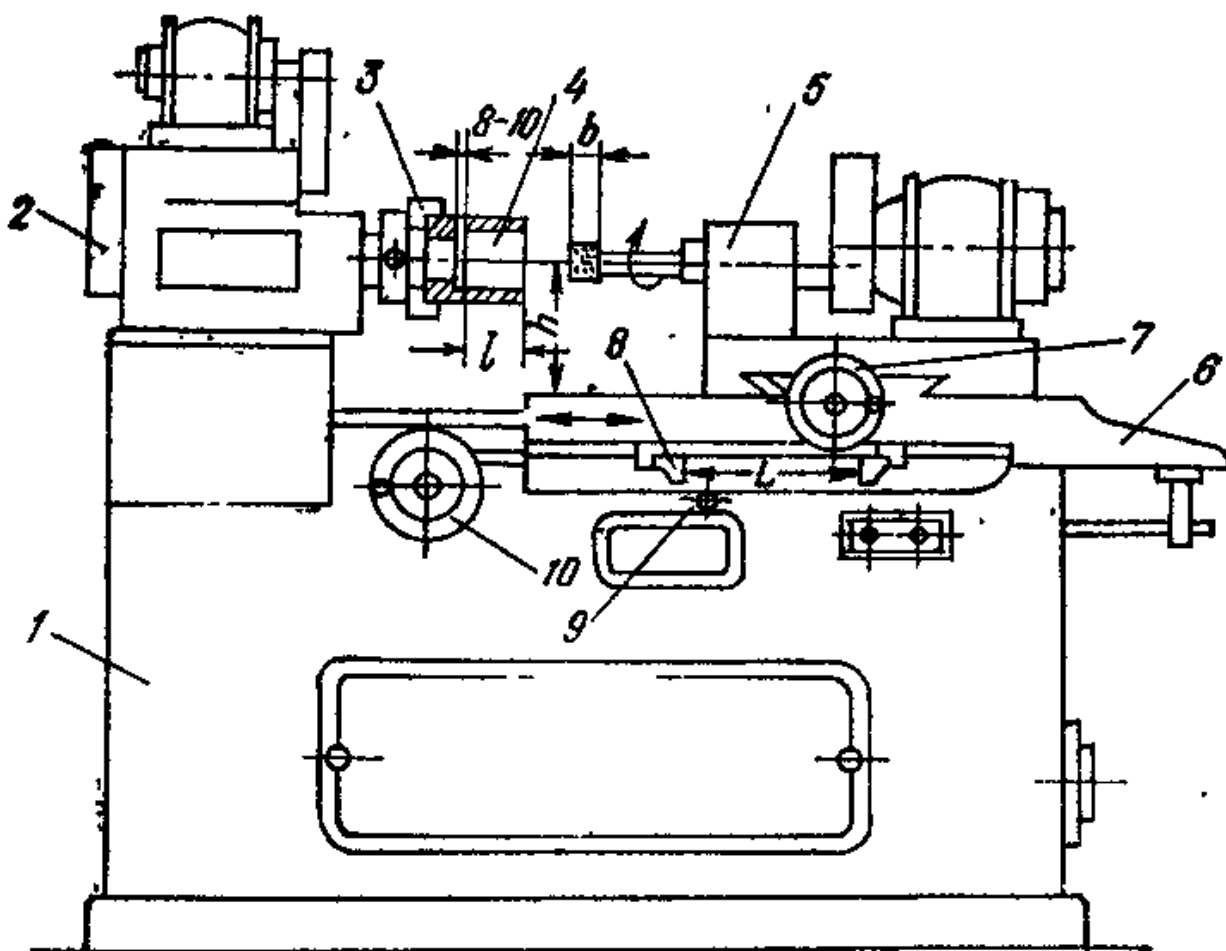
1-rasm. Ichki yuzalarni jilvirlash stanogining umumiy kurinishi:
