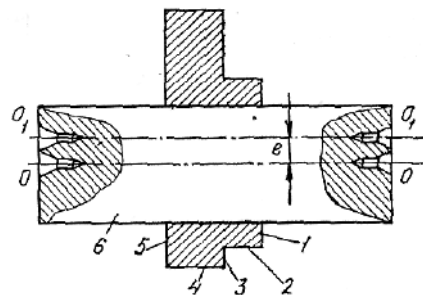
73-рasm. Доирaviй эксцентрик юзаларни ишлашда заготувканинг ишлаш схемаси.
