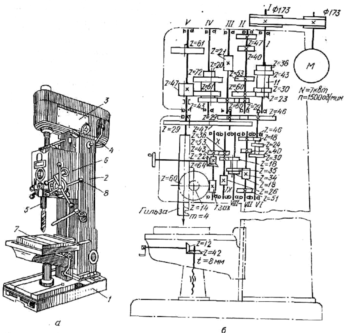
76-расм. 2А150 маркали пармалаш станогини кўриниши (а) ва кинематик схемаси (б)
