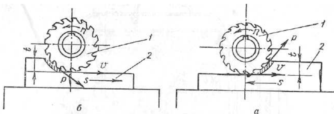
79-рasm. Фрезалаш усуллари: а — қарши фрезалаш; б — фўлаки фрезалаш.
