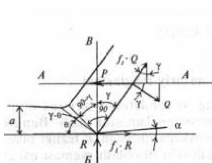
4.4-rasm. Keskich tig'iga ta'sir etuvchi kuchlar sxemasi.
