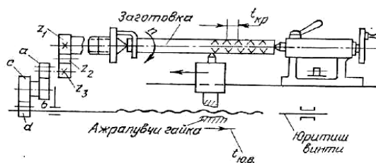
75-рasm. Токарлик станокда иппинделдан юргизиш винтига ҳаракат узатиш схемаси.
