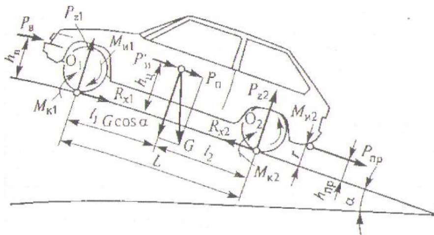
-- rasm . Balandlikka chiqayotgan avtomobilga tezlanish vaktida ta'sir etayotgan kuchlar.
