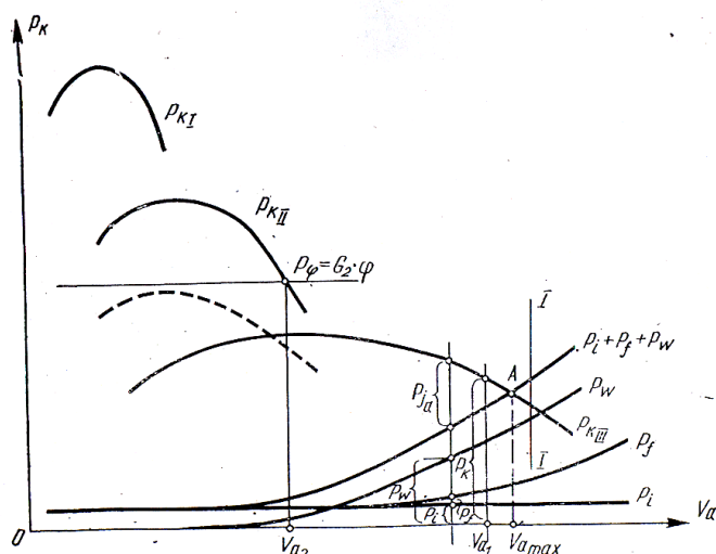
21.1-rasm. Kuchlar muvozanati tenglamasi va uni yechilishi.
