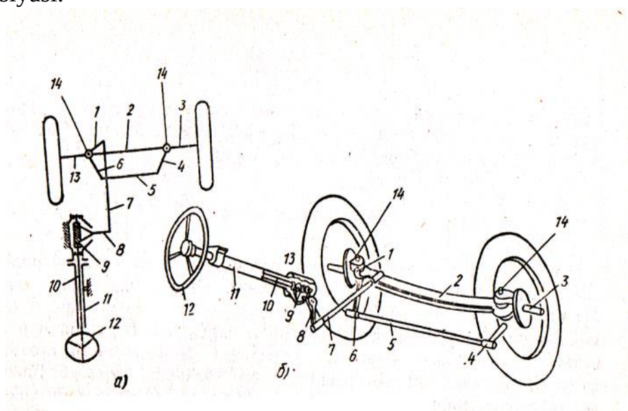
7.1-rasm. Avtomobilning burilish tizimini tasviriy chizmasi va rul trapetsiyasi.
