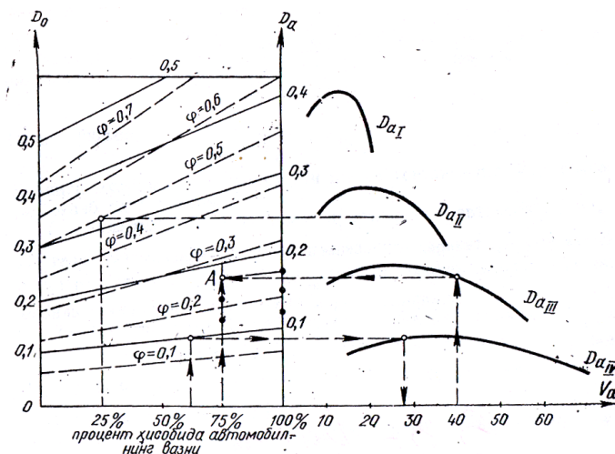
5.1-rasm. Avtomobilning dinamik pasporti grafigi.
