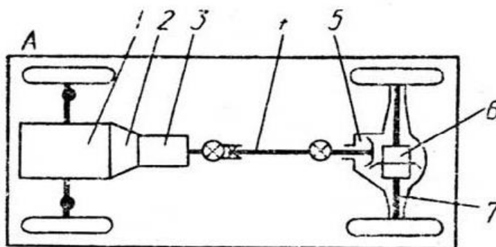
1.1-rasm. Avtomobilning umumiy tuzilishi chizmasi.
