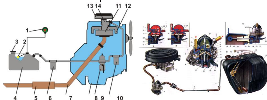
8.1-rasm. Karbyuratorli dvigatelning yonilg'i bilan ta'minlash tizimi asboblarning joylashish chizmasi .
