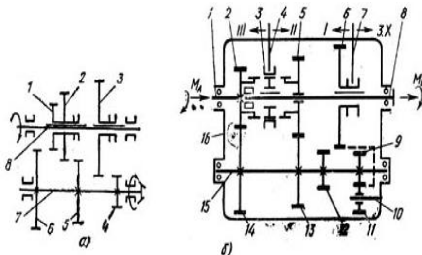
4.3-rasm. Uzatmalar qutisining tasviriy chizmasi.
