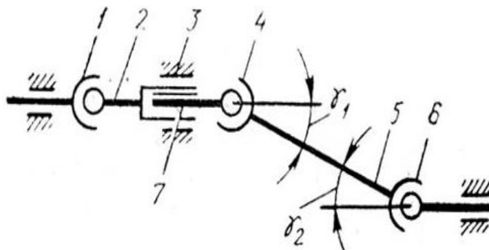
5.1-rasm. Kardan uzatmaning soddalashgan tasviriy chizmasi.
