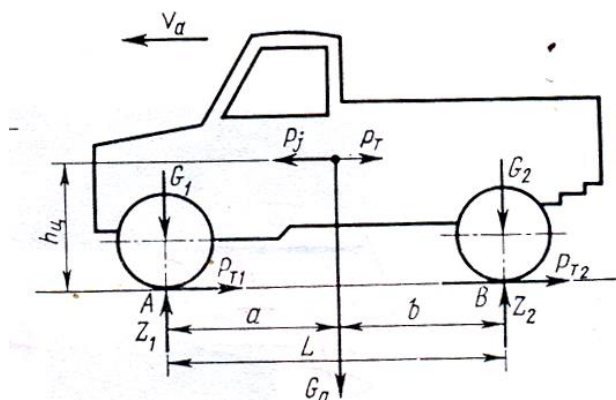
11.1-rasm. Avtomobilning yelkanlik markazining koordinatalari.
