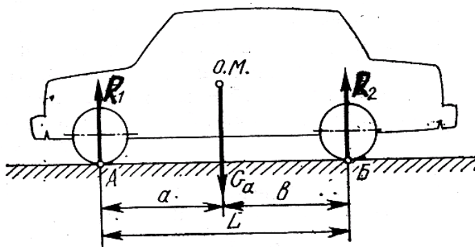
21.2-rasm. Gorizontal yo'lda harakatsiz turgan avtomobilga ta'sir qiluvchi og'irlik va reaksiya kuchlari.
