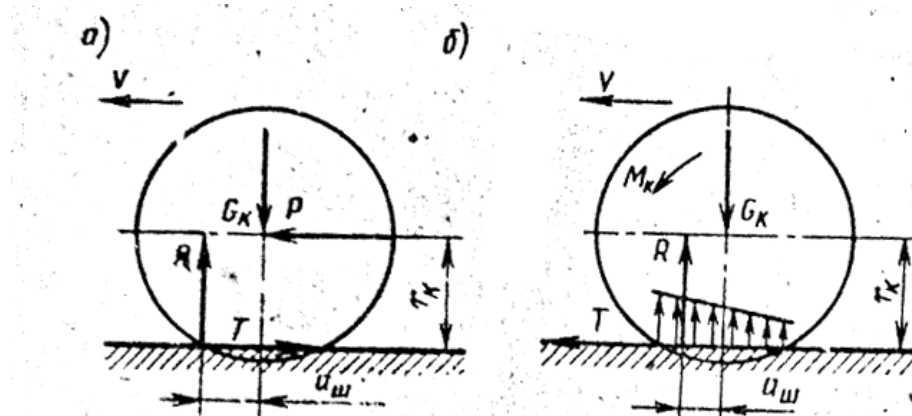
20.2-rasm. Yetaklanuvchi va yetakchi g'ildiraklarga ta'sir etuvchi kuchlar va momentlar: a-etaklanuvchi g'ildirakka ta'sir etuvchi kuchlar va momentlar, b-etakchi g'ildirakka ta'sir etuvchi kuchlar va momentlar.
