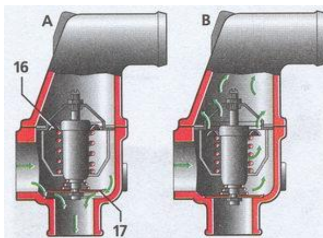
6.2-rasm. Termostatlarning sxemalari: a-suyuqlik termostati; b-qattiq to'ldirgichli termostat; I va IV-termostatlar ochiq; II va III-termostatlar yopiq; 1-suv nasosining korpusi; 2-suyuqlik balloni; 3 va 13-shtoklar; 4-qistirma; 5 va 15-termostatlarning klapanlari; 6 va 16-qaynoq suyuqlikni chiqarish patrubkalari; 7 va 18-termostatlarning korpuslari; 8-kronshteyn; 9-termostat balloni; 10-qattiq aralashma; 11-diafragma; 12-yo'naltiruvchi vtulka; 14-qaytargich prujinasi; 17-klapan koromislosi; 19-bufer; 20-kiritish o'tkazgichi.
