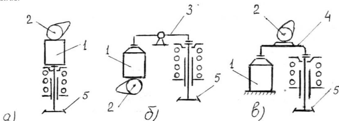
5.5-rasm. Hidrokompensatorni joylashtirish usullarining sxemalari:
