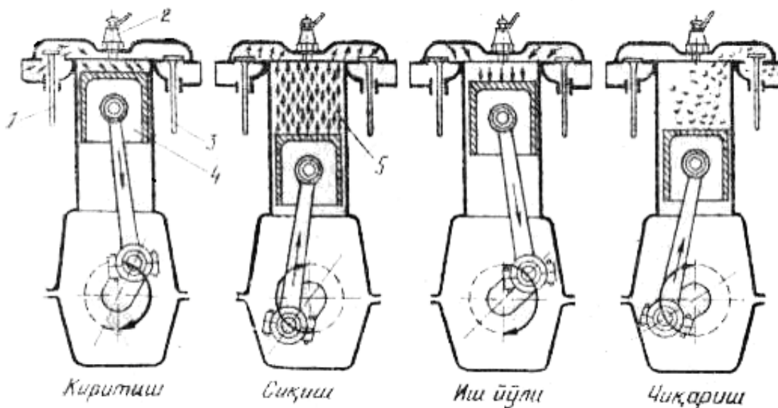
3.3-rasm. Bir tsilindrli karbyuratorli dvigatelning ish tsikli. 1-kiritish klapani, 2-yondirish shami (svecha), 3-chiqarish klapani,
