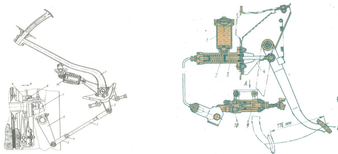
11.6-rasm ilashish muftasining boshqarish yuritmalari. a- mexaniq boshqarish yuritmasi; b-gidromexanik boshqarish yuritmasi;
