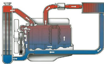
6.1 – rasm. Suyuqlik bilan sovutish tarmogʻining ishlash tasviri.
