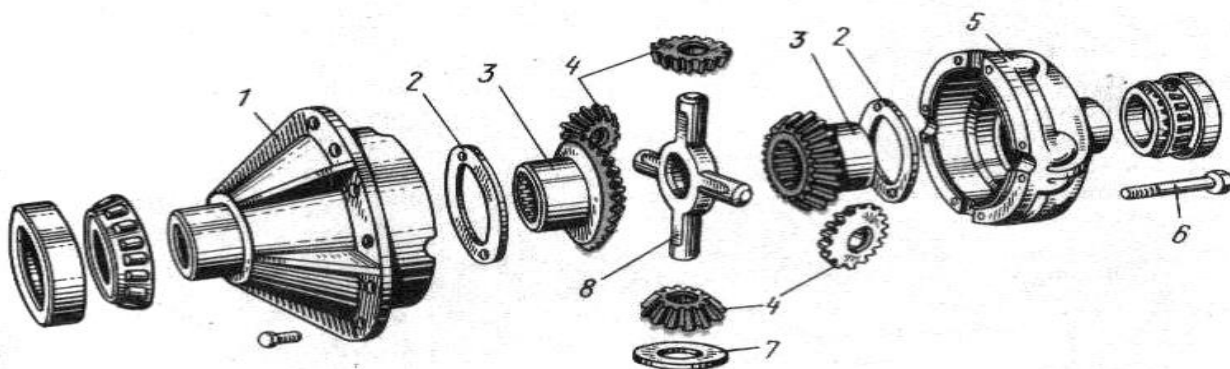
14.5-chizma Konus shesternyali g'ildiraklararo simmetrik differentsialning shakli.
