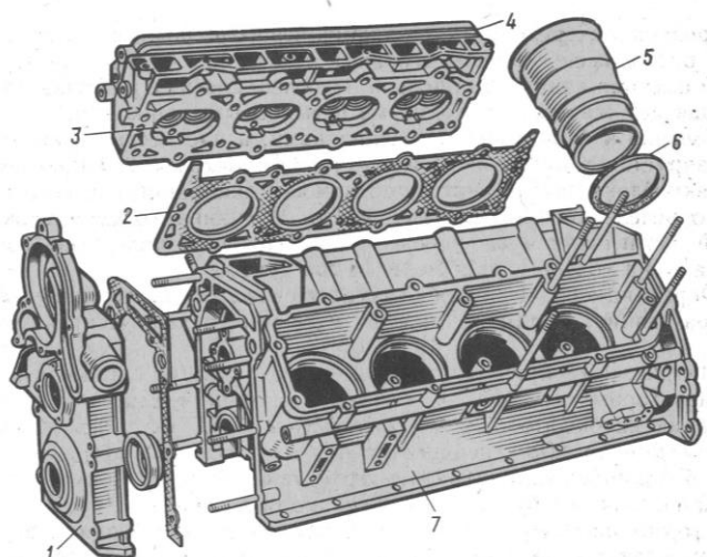
4.5-chizma. V-simon dvigatelning blok karteri va tsilindrlar bloki kopkog'i. 1- tishli g'ildirklarni taqsimlash blok qopqog'i, 2- blok qopqog'i qistirmasi, 3-yonish kamerasi, 4-tsilindrlar bloki qopqog'i, 5-tsilindrlar gilzasi, 6-zichlovchi halqa, 7-blok-karter.
