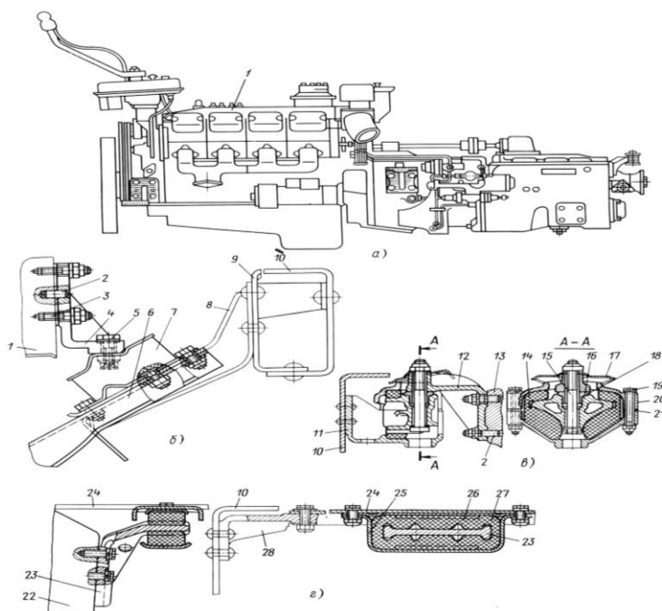
4.6-rasm. KamAZ-5320 avtomobili dvigatelining maxkamlanishi: a-dvigatel; b-old tayanch; v-orqa tayanch; g-ushlab turuvchi tayanch; 1-tsilindrlar bloki; 2-shtift; 3-shpilka; 4,8,23 va 28-kronshteynlar; 5,15 va 19-boltlar; 6-tortgich; 7,14 va 27-rezina yostiqlar; 9-ustun; 10-rama lonjeroni; 11-orqa tayanch kronshteyni; 12-dvigatel kronshteyni; 13-maxovik karteri; 16-barmoq; 17-himoya qalpog'i; 18-vtulka; 20-qopqog; 24-rostlovchi qistirma; 22-uzatmalar qutisi karteri; 24-ko'ndalang list; 25-yostiqlarning oboymasi; 26-yostiqlarning nakladkasi.
