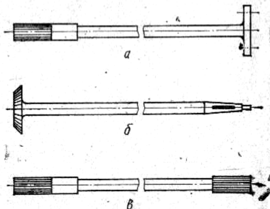
14.6-rasm. Avtomobillarning yarim o'qlari
