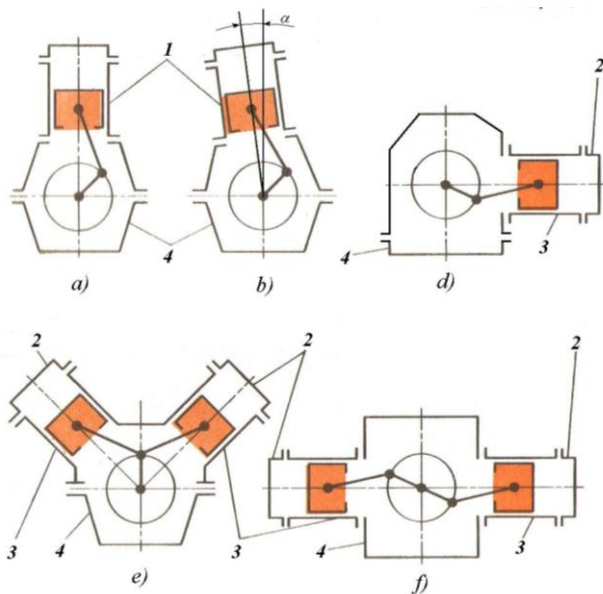
4.1-rasm. Dvigatel tsilindrlarining joylanish sxemasi
