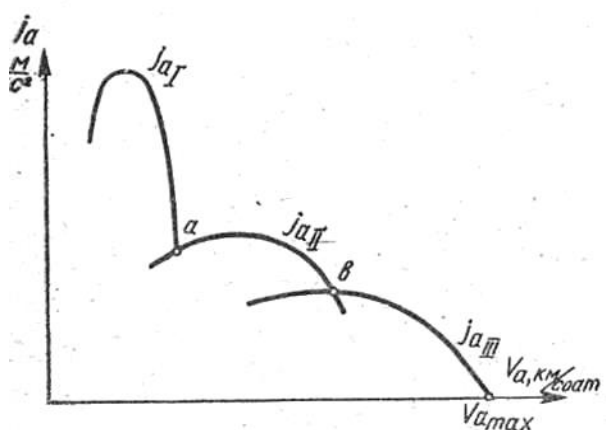
21.5-rasm. Avtomobilning tezlanish grafigi
