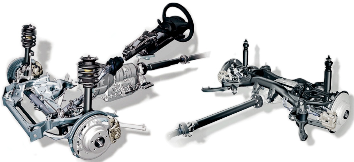
15.6-rasm. Mustakil osma turlari.
