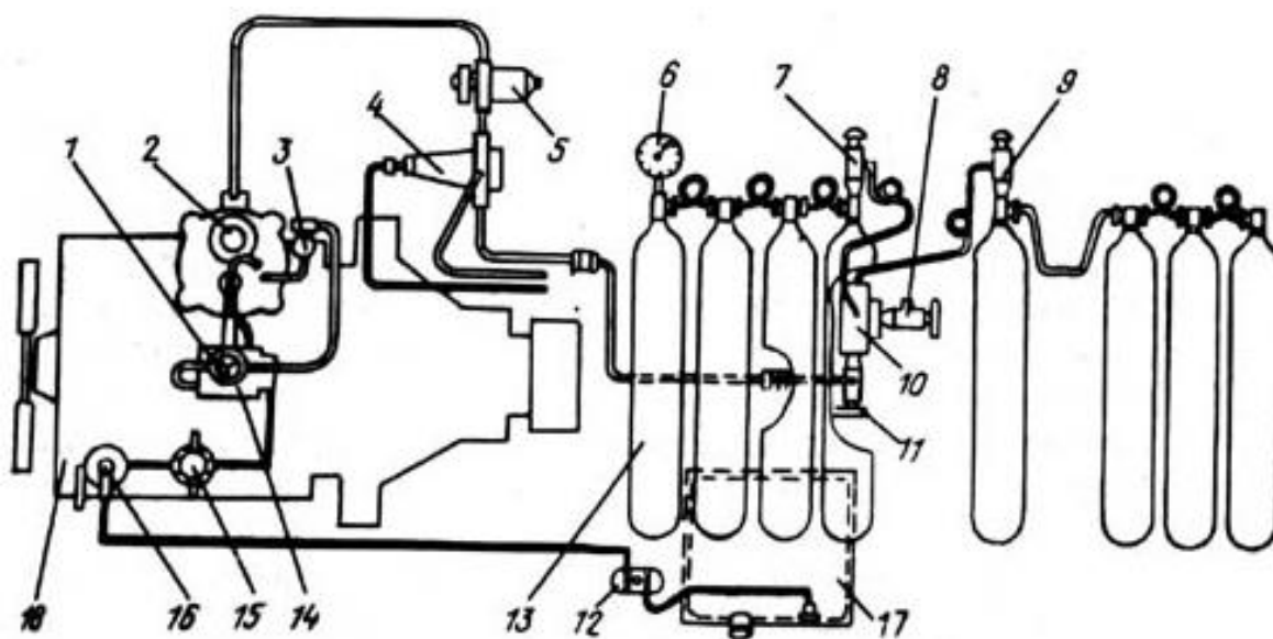
3.7-rasm. Yuqori bosimli gaz ballonda ishlovchi ZIL-43610 avtomobil dvigatelining gaz balonli ta'minot uskunasi umumlashgan chizmasi.
