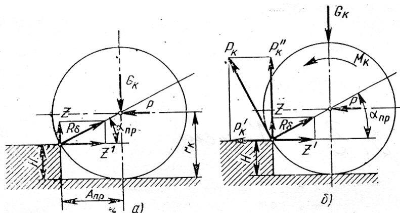
25.2-rasm. G'ildiraklarning to'siqdan o'tishi. a) yetaklanuvchi oldingi g'ildirak. b) yetakchi orqa g'ildirak.
