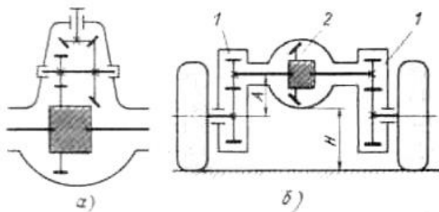
14.2-rasm. Qo'shaloq asosiy uzatmalarning turlari:
