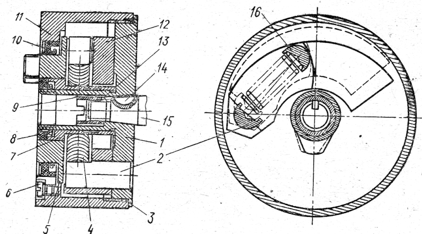
10.6–rasm. Yonilg'ini ilgarilatib purkovchi avtomatik mufta.
