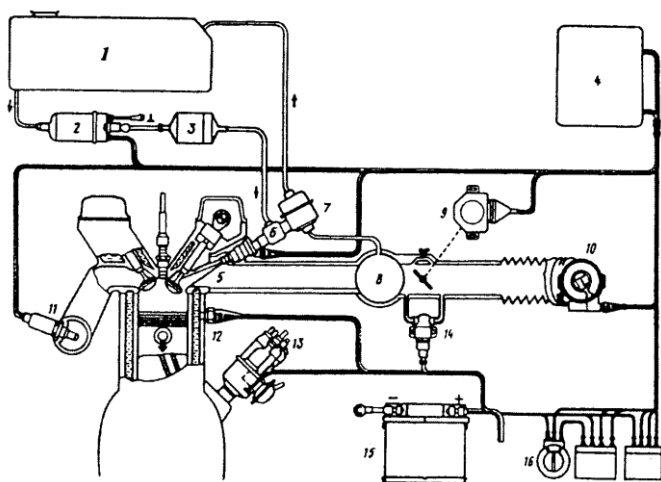
8.6-rasm. Taqsimlangan purkash tizimi. 1-yonilg'i baki; 2-elekt nasos; 3-moyni tozalash filtri; 4-elektronli boshqarish bloki; 5-elektromagnitli forsunka; 6-haydash magistrali; 7-reduksion klapan; 8-kiritish quvuri yo'li; 9-drossel zaslonkasi vaziyati datchigi; 10-havo sarfi ulagichi; 11- \lambda -zond; 12-harorat datchigi; 13-o't oldirish taqsimlagichi; 14-qo'shimcha havo rostlagichi; 15-akkumulyator; 16-o't oldirish qulfi.
