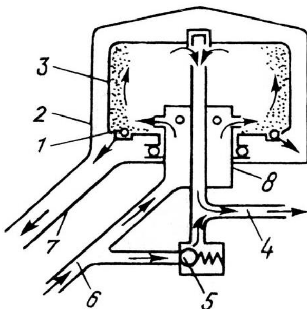
3.4-rasm. Tsentrafuganing soddalashgan chizmasi.
