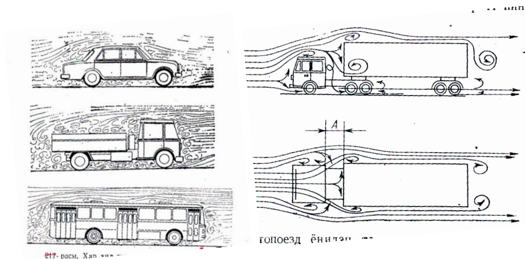
20.7-rasm. Har xil turdagi avtomobillarga havo oqimini ta'siri
