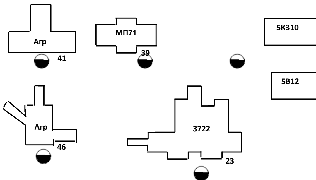
7.3-rasm. Metall kesish dastgohlari va ish joylarining shartli grafik belgilari (davomi)
