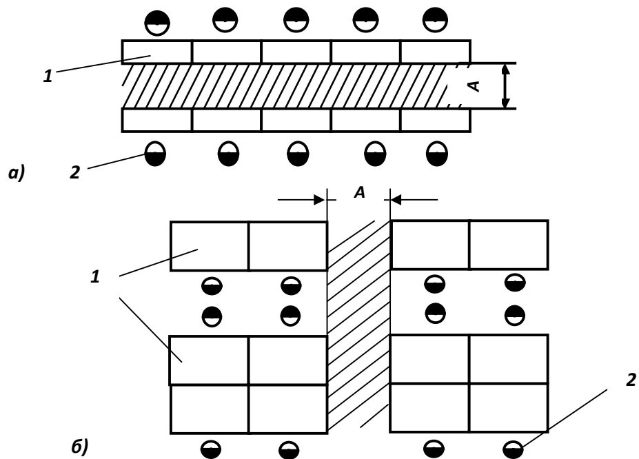
10.9-rasm. Verstaklar orasida vo'lak va vo'lkalarning
