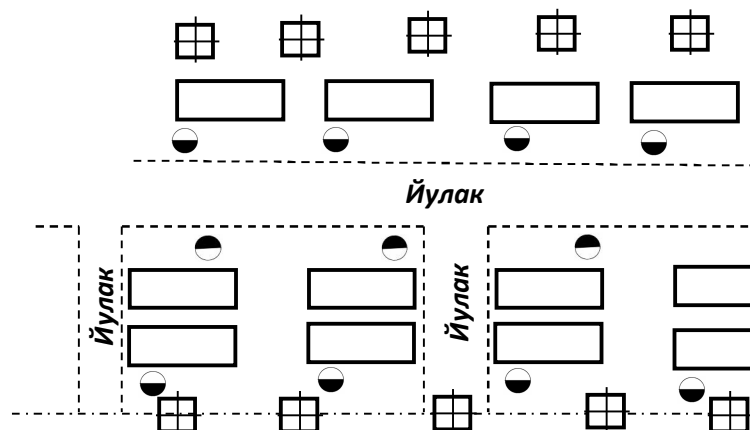
7.17-rasm. Dastgohlarni bir prolyot ichida bir bo'ylama va uch ko'ndalang yo'laklarda joylashtirish
