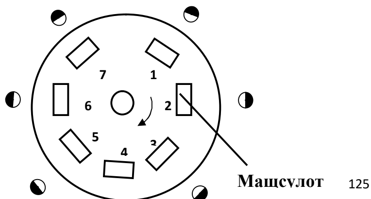
10.6-rasm. Dastgohlarni umumiy yig'ish uchun qadamli konveyer
