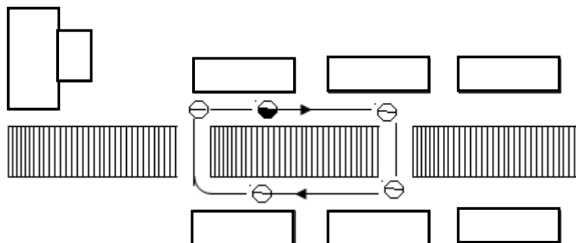
7.26-рasm. Ko'p dastgohli xizmat ko'rsatishda rolyang atrofida dastgohlarni ikki qator joylashtirish
