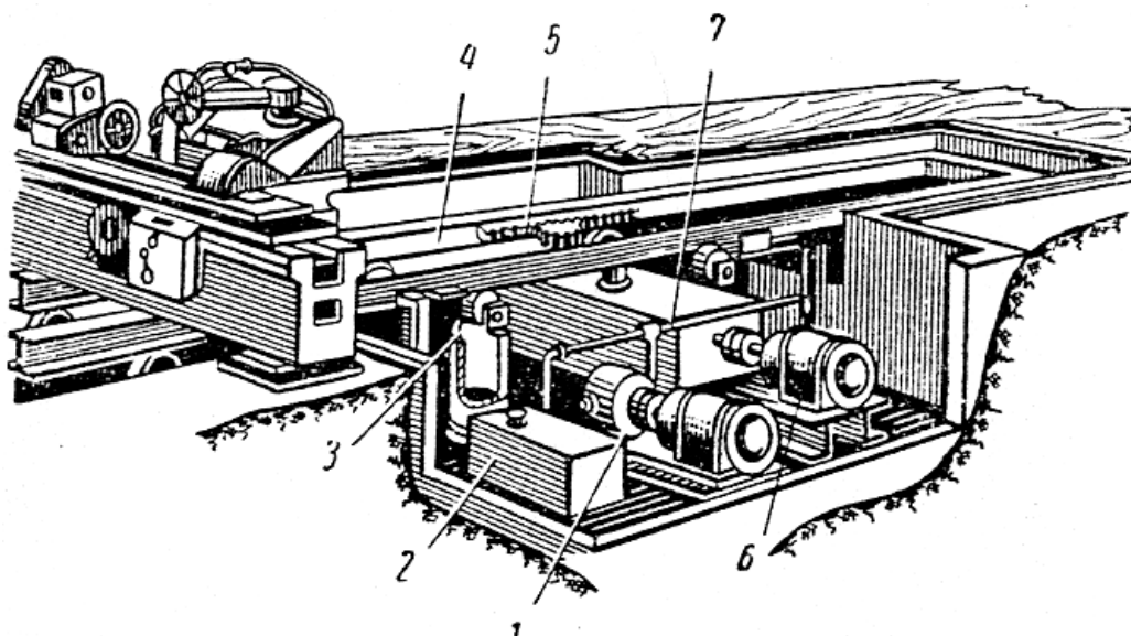
10.6-rasm. Dastgohlarni umumiy yig'ish uchun qadamli konveyer
