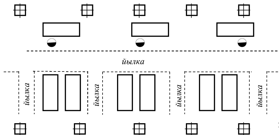
7.18-rasm. Dastgohlarni prolyot bo'yicha ikki qatorli parallel bo'ylama yo'laklarda joylashtirish
