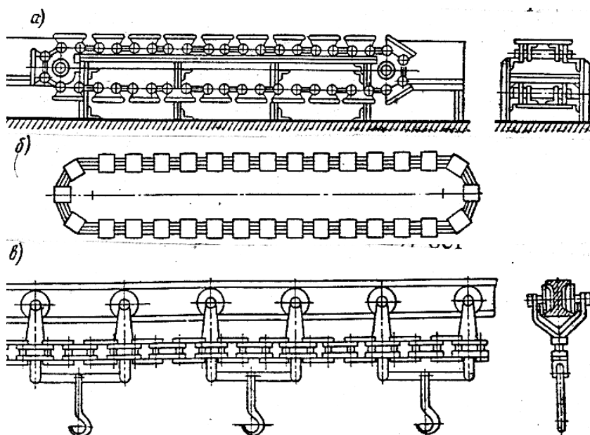
10.5-rasm. Yig'ish ishlari uchun konveyerlar sxemasi
