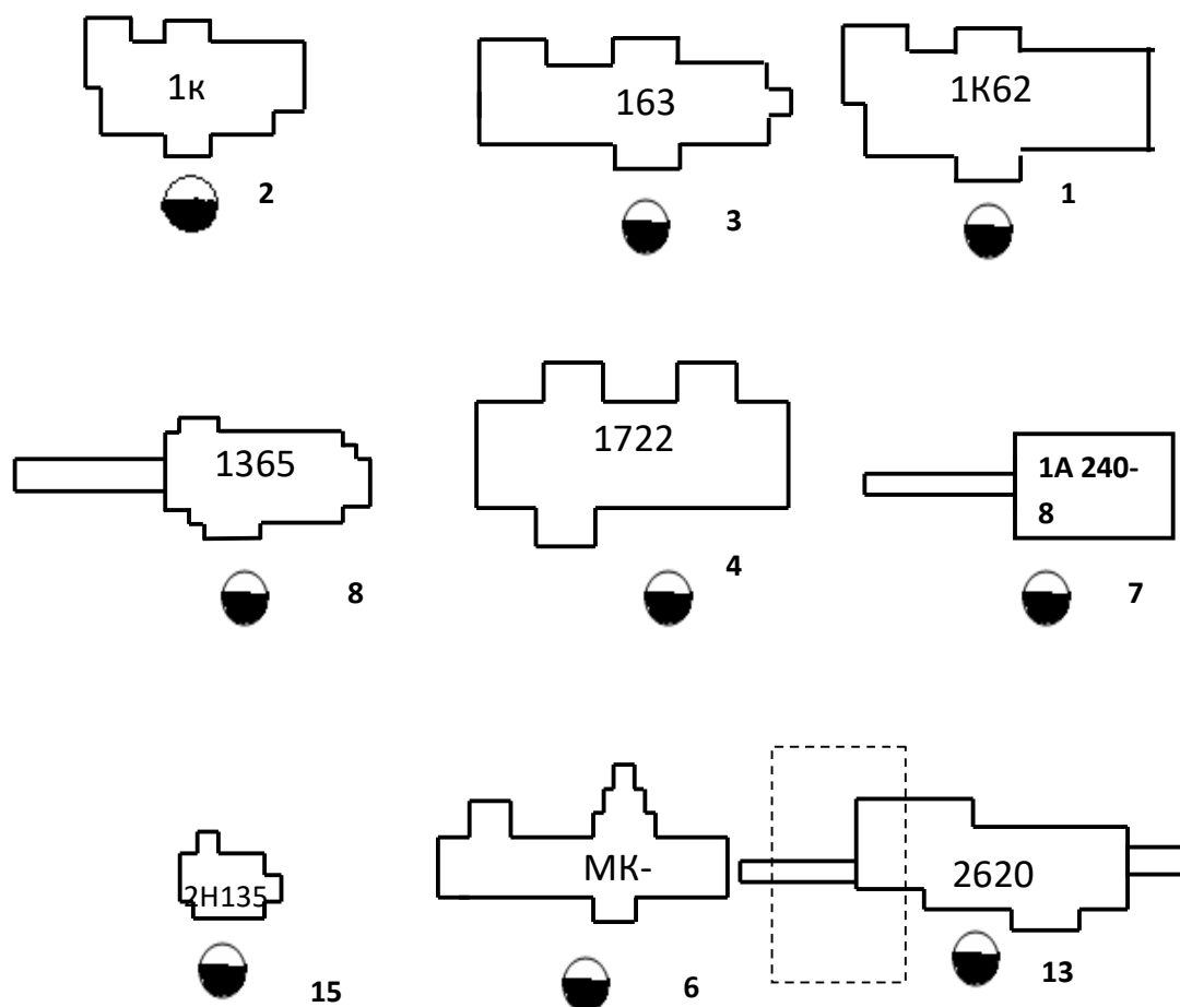
7.3-rasm. Metall kesish dastgohlari va ish joylarining shartli grafik belgilari
