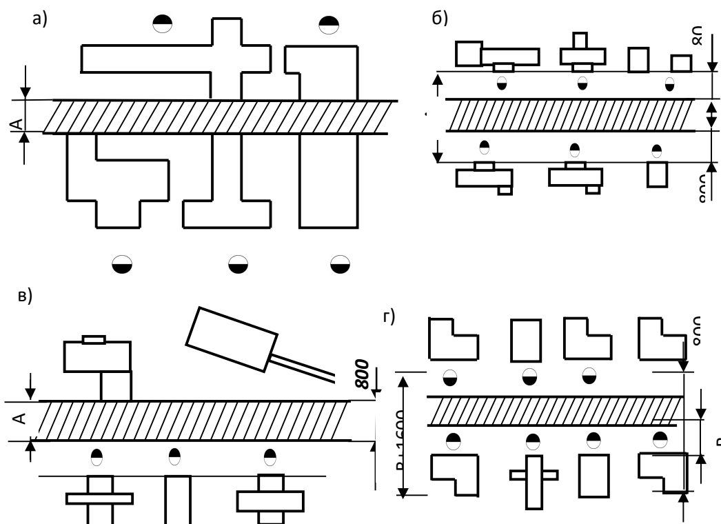
7.14-rasm. Dastgohlar orasidagi yo'lak kengligi, liniya dastgohlari bilan osma va yer usti konveyerlari orasidagi masofalar
