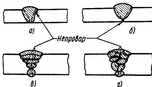
4.9-rasm. Pishmagan (etilmagan) joylar:
