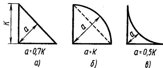
4.2-rasm. Valikli choklarning asosiy konstruktiv elementlari: a – normal (me'yordagi), b – qavariq, v – boshiq
