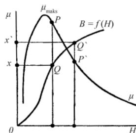
5.4- rasm. Ferromagnit material uchun B va \mu ning H ga bog'liqligi.
