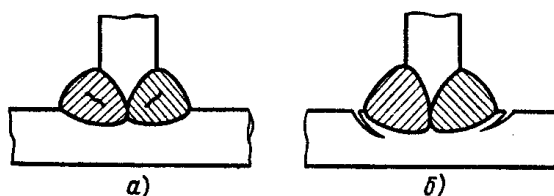
4.10-rasm. Payvand chok va birikmalardagi yoriqlar:
