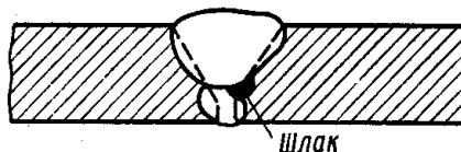
4.8-rasm. Ko'p qatlamli chokda uchning kesilishi bo'yicha shlakli kirishmalar.
