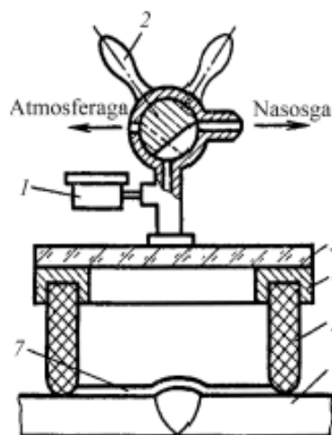
7.5- rasm. Zichlikni vakuum kamerasi yordamida nazorat qilish sxemasi:
