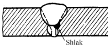
8- rasm. Ko'p qatlamli chokda uchning kesilishi bo'yicha slagli kirishmalar.
