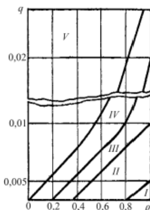
18- rasm. Nuqsonning real (haqiqiy) va potensial xavfliligini belgilovchi q va p parametrlarga bog'liq holda payvand choklari nuqsonlarining sinflari (I, II, III, IV, V).
