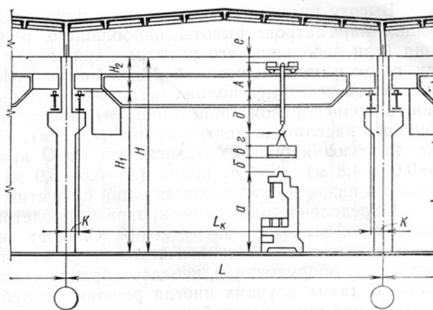
5.2-rasm. Opaliqning parametrini aniqlash uchun bir qavatli bino qirqim sxemasi.
