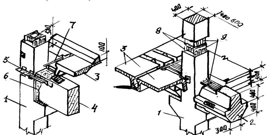
Rasm 19. Orayopmalarni rigellarga (to'sinlarga) o'rnatish uzellari a – to'g'riburchakli rigellarga, b – polkali rigellarga:
