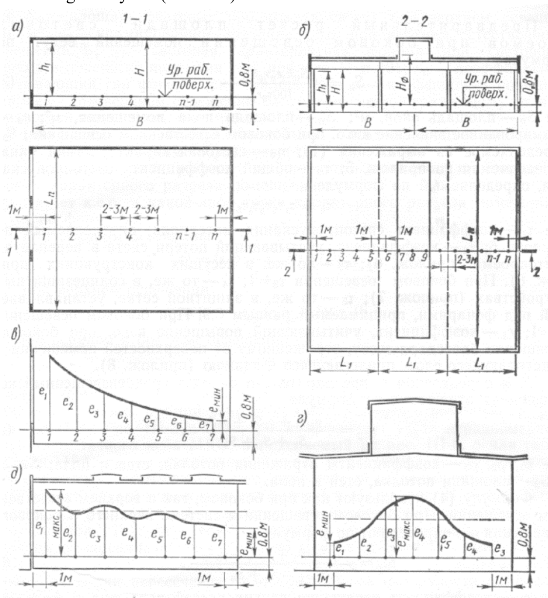
3.1 - rasm. Xonalarning tabiiy yoritilishini hisoblash uchun.
