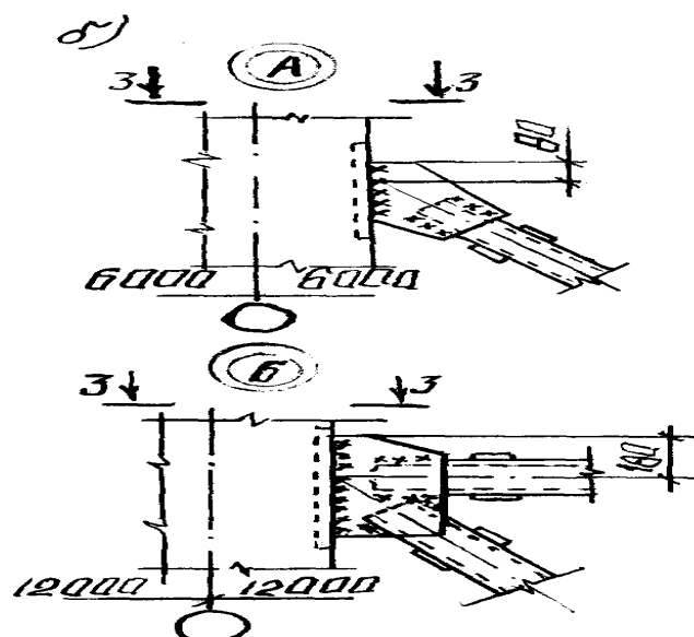
Rasm 16. Temir beton ustunlar orasidagi bog'lovchilar a – umumiy ko'rinishi, b – bog'lovchilarni ustunlarga mahkamlash detali; 1 – ikssimon bog'lovchilar, 2 – portal bog'lovchilar
