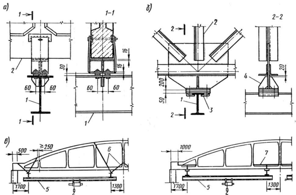
7.12 rasm. Stropila konstruktsiyasiga osma kranning yo'lini mustahkamlash.
