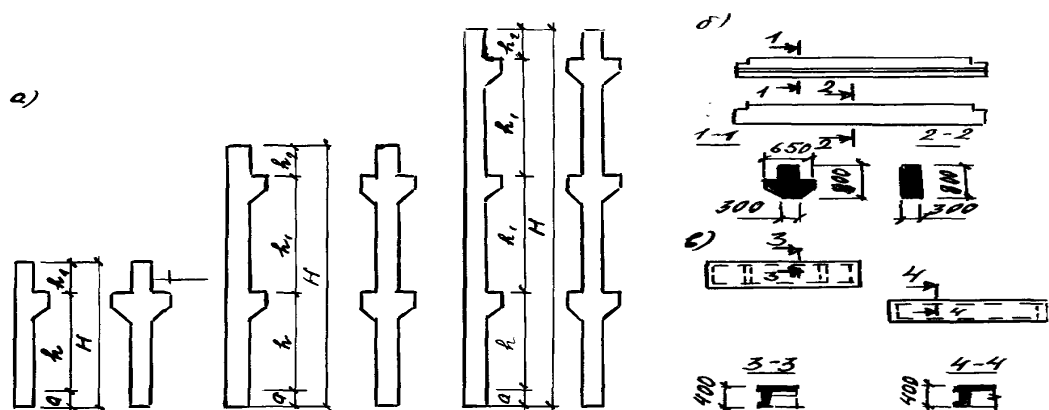
Rasm 18. Orayopma to'sini tayanadigan ko'p qavatli ishlab chiqarish binolarining unifikatsiyalangan yig'ma temirbeton elementlari: a – ustunlar, b – rigel (to'sin), v – yopma plitalar
