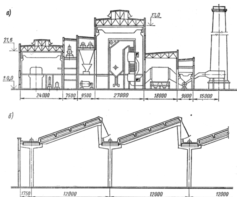
5.2-rasm. Opaliqning parametrini aniqlash uchun bir qavatli bino qirqim sxemasi.
