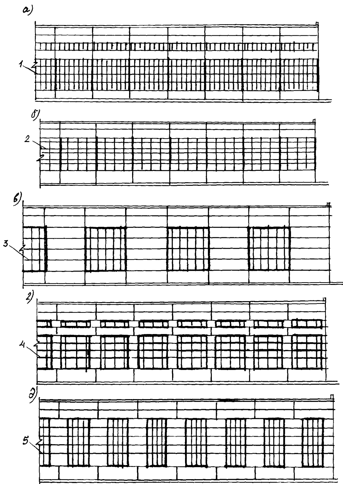
Rasm 21. Bir qavatli binolar devorlari qirqimidan variantlar
