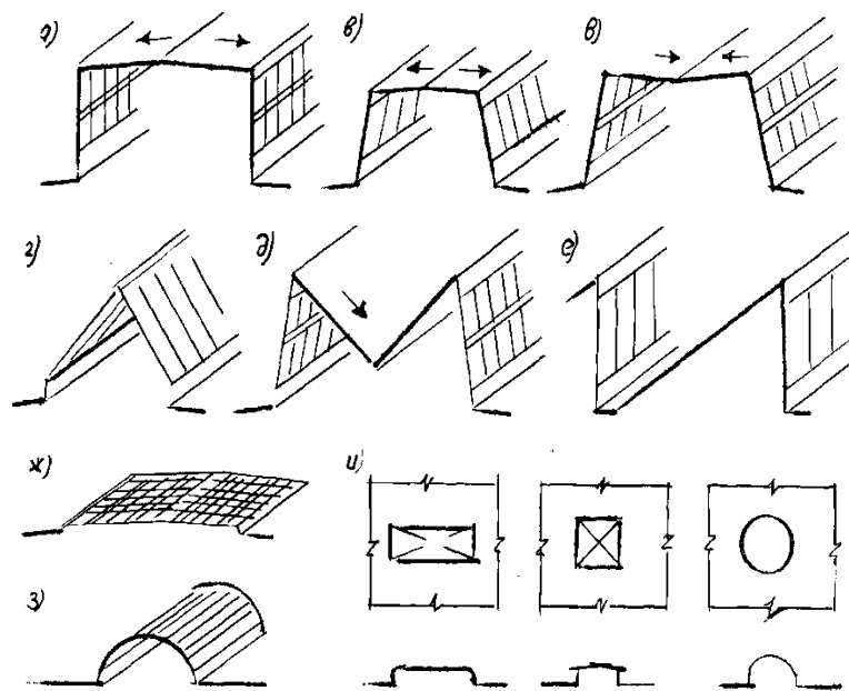
Rasm 30. Yorug'lik (yorug'lik+aeratsiya) fonarlarini asosiy turlari a – to'g'riburchakli, b,v – trapetsiyasimon, g – uch burchakli, v – M- shaklida, ye – shedasimon, j-i – zenit
