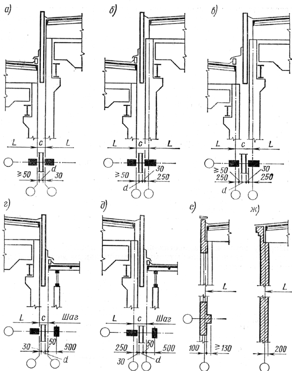
4.3 rasm. Bir qavatli bino elementlarini biriktirish va enlama rejalar o'qlariga bog'lash.
