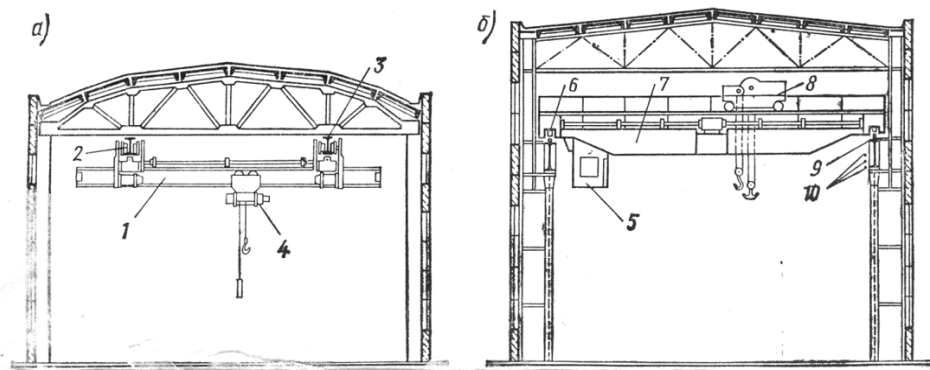
2.4- rasm. Osmo va ko'priksimon kranli binolar.
