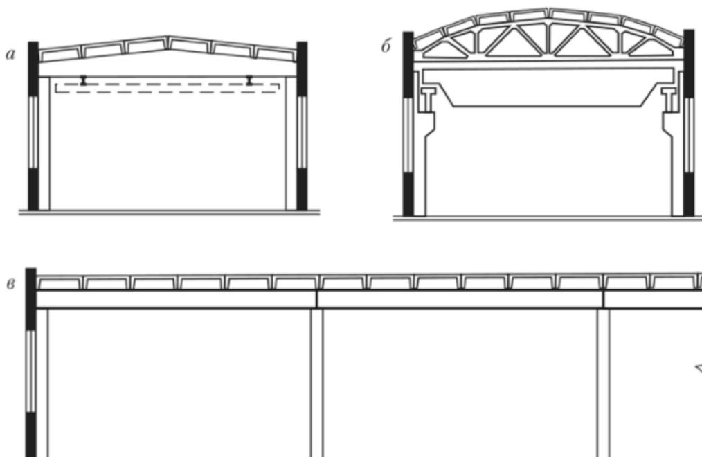
Rasm-1. Bir qavatli sanoat binolariing asosiy ko'rinishlari
