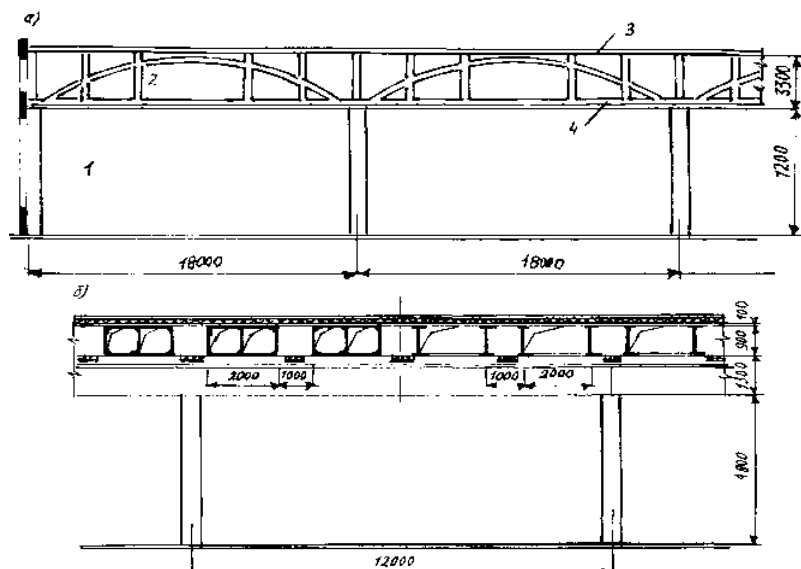
Rasm 8. Bir qavatli universal binolar
