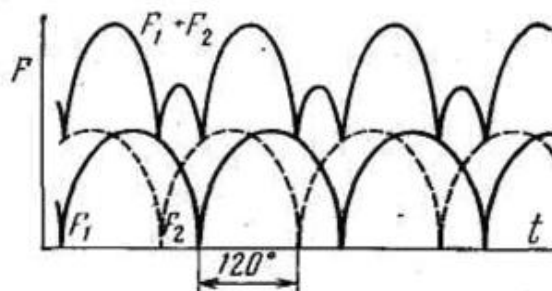
3-rasm. «Fazasi bo'lingan» sxema bilan ulangan lampalarning yorug'lik oqimini lipillashini kamayishi diagrammasi.
