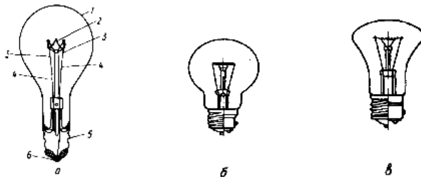
1-rasm. Umumiy qo'llaniladigan cho'g'lanma chiroqlarning tuzilishi:
