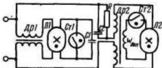
1-rasm. Lyuminescent lampalarni «fazalari bo'lingan» sxema bilan ulash
