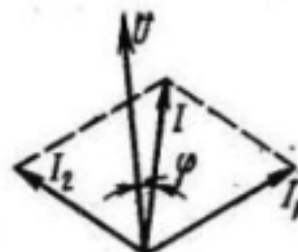
2-rasm. Lampalarni «fazasi bo'lingan» sxema bilan ulangandagi toklarning vektor diagrammasi.
