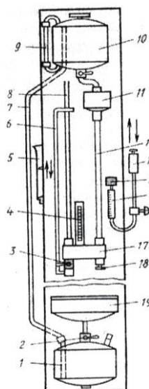
5.1-расм. Жиклёрнинг ўтказувчанлигини текширадиган НИАТ-528 русумли асбоб. Жиклёрни текшириш тартиби
