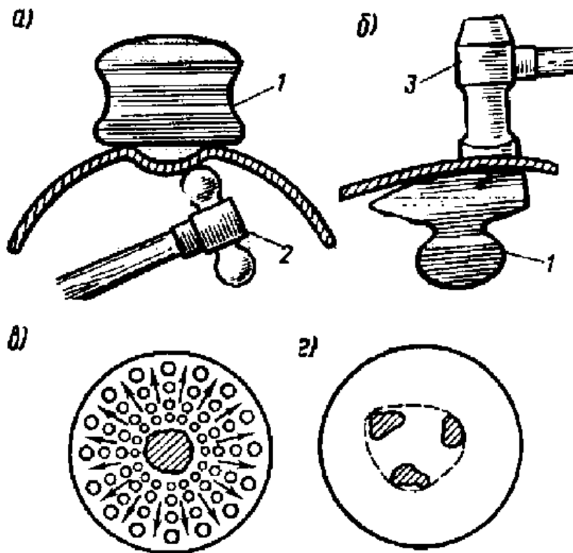
9-rasm. Pachoqni chiqarish va tekislash shakli: a-ushlagich yordamida pachoqni chiqarish; b-ushlagich yordamida to'g'rilash; v-bir pachoqni bartaraf etish; g-bir necha pachoqni bartaraf etish.
