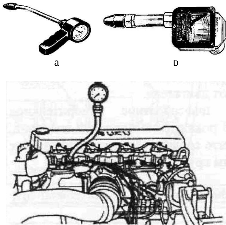
14-Rasm. Manometrli (a) va o'zi yozuvchi (b) kompressometrlar hamda Isuzu avtomobili dvigatelining kompressiyasini o'lchash shakli (s).
