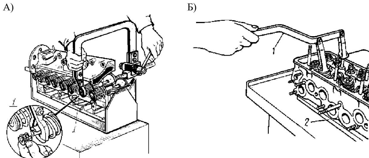
7.24-rasm. TSilindr kallaklarini bo'laklarga ajratish shakli: 1-klapan birikmasini yechish moslamasi; 2-klapanlarni harakatini chegaralovchi taglik
