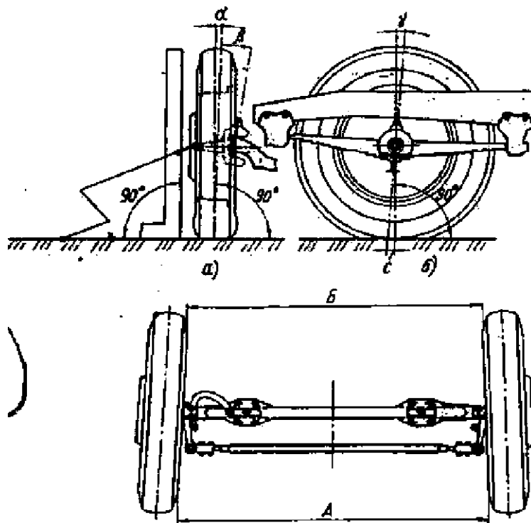
52-rasm. Boshqariladigan g'ildiraklarni o'rnatish shakli: a-og'ish \alpha va shkvorenning ko'ndalang qiyalik R burchaklari; b-shkvorenning bo'ylama qiyalik u burchagi; v -g'ildiraklarning yaqinlashuv masofasi
