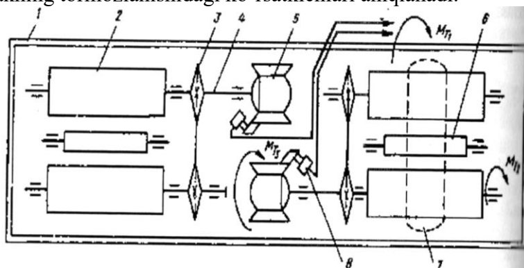
3.2-rasm. Kuch yuritmalı tormoz stendining sxematik ko'rinishi. 1-rama; 2-rolık; 3-zanjirli uzatma; 4-val; 5-motor-reduktor; 6-blokirovkalovchi rolik; 7-avtomobil g'ildiragi; 8-bosim datchigi.
