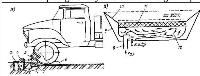
4-shakl: Moslama va infra qizil nur tarqatuvchi garelka shakli. 1-quduqcha; 2-gaz o'tkazgich; 3-jo'mrak; 4-shlanga; 5-gaz garelkasi; 6-yo'naltiruvchi; 7-tayanch; 8-gaz etkazuvchi shtutser; 9-garelka korpusi; 10-nurlatuvchi korpusi; 11-nurlatgich; 12-aralashtirish kamerasi.
