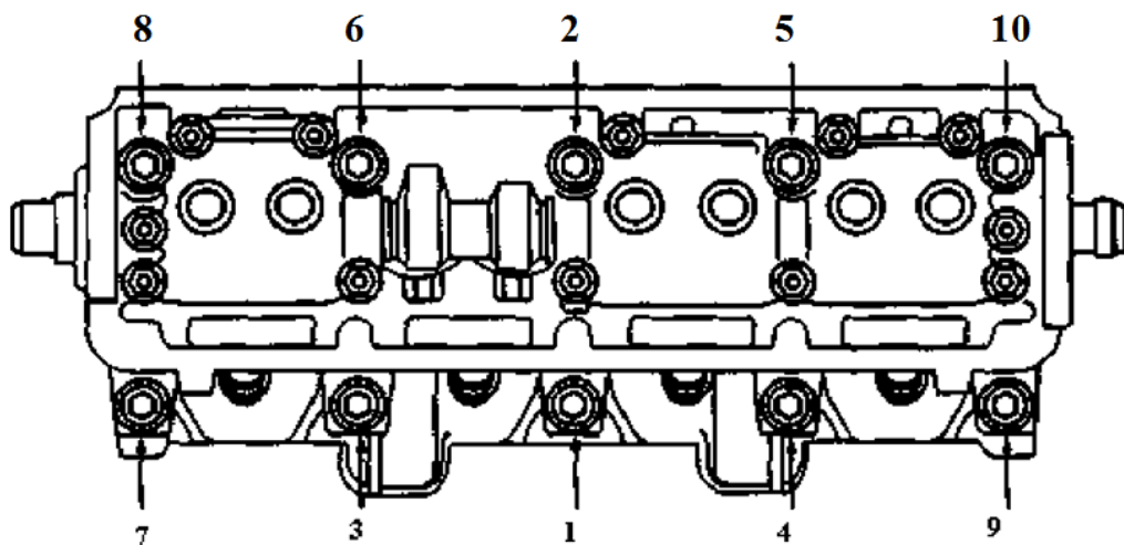
16-расм. Нексия SOHC-двигателларининг цилиндр каллаклари гайкаларини маҳкамлаш кетма-кетлиги
