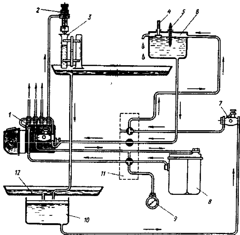
38-rasm. Yonilg'i nasoslrini tekshirish jihozining ishlash shakli: 1-yuqori bosimli yonilg'i nasosi, 2-etalon forsunka, 3-menzurka, 4-yonilg'i sathini ko'rsatkich, 5-termometr, 6, 10-yonilg'i bakchalari, 7-jihozning yonilg'i haydash nasosi, 8-filtr, 9-manometr, 11-kranlar, 12-yonilg'ini to'plovchi vanna
