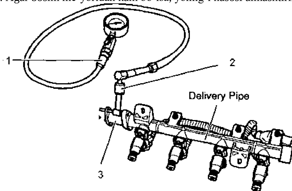
35-rasm. Yonilgʻi taʼminot tizimidagi bosimni tekshirish: 1-manometri; 2- ulagich; 3-quvuroʻtkazgich.
