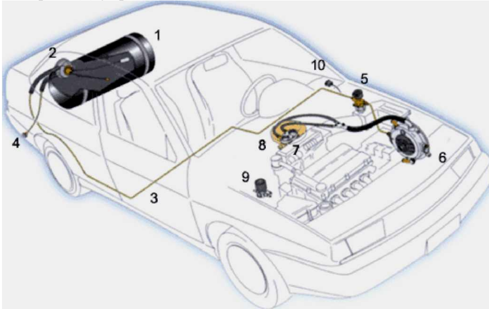
42-rasm. Karbyuratorli avtomobillarning uchinchi avlod gaz-ballon jihozlarning ko'rinishi: 1-ballon; 2-mul'tiklapan; 3-yuqori bosim gaz magistrali; 4-gazni to'ldirish moslamasi; 5-gaz klapani; 6-reduktor-bug'latgich; 7-dozator; 8-gaz va havoni aralashtirgich; 9-benzin klapani; 10-yonilg'i turlarini ulagich.
