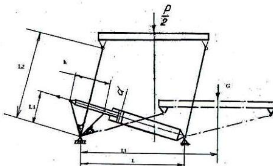
13-rasm. Richagli gidravlik ko'targichning xisobiy sxemasi.
