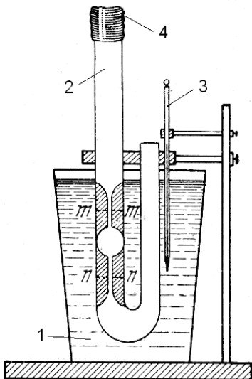
1.2-rasm. Kapillyar viskozimetrning ish jarayoni
