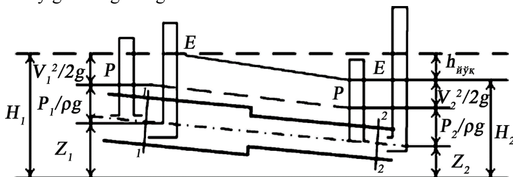
Расм15. –Реал суюклик учун Бернулли тенгламасининг
