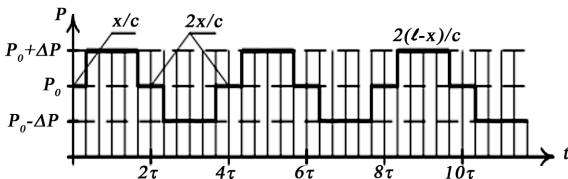
Рисм 28. – қопқокдан x = 0,5l масофада босим
