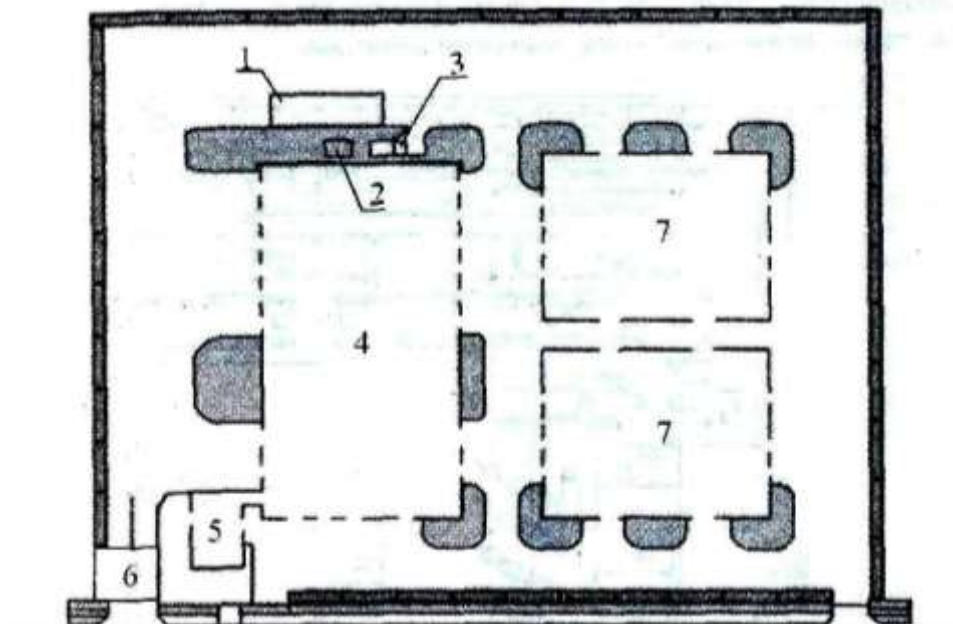
2.40-rasm. Katta sinfdagi 300 ta avtobus uchun ATK ning bosh rejasi:
