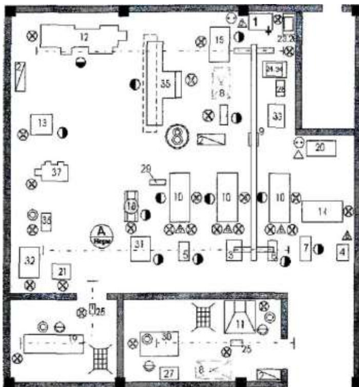
2.14-rasm. "Maxsustrans" avtokorxonasi agregat-mexanik ustaxonasining rejasi.
