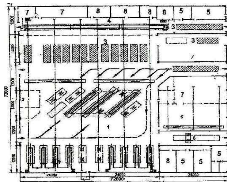
35-rasm. 250 ta KamAZ avtopoyezdlad ucun yuk ATK sining rejasi :
