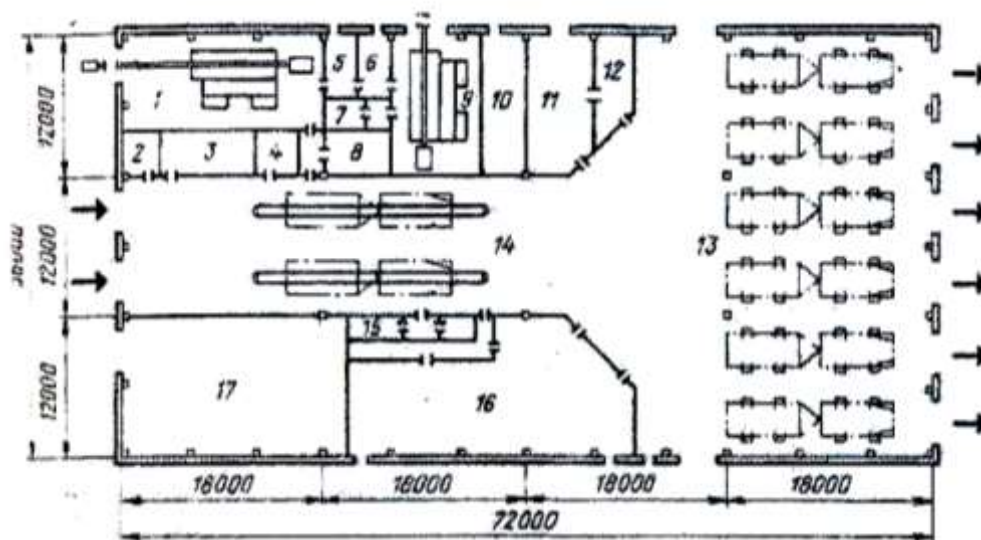
2.38-rasm 300 yuk avtomobili uchun ATK ning KKK va bo'yoqchilik ustaxonasi binosimng rejasi:
