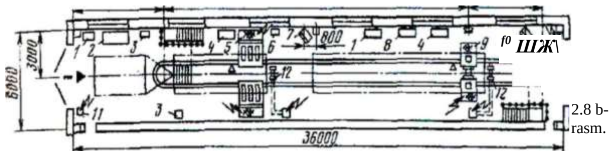
Автопоезdlар ТSh-1 ташхисlash mintaqasi rejasl:
