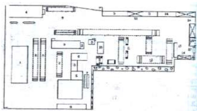
2.54-rasm. Olmaliq tog'- metallurgiya kombinati avtotransport boshqarmasiiring 3-avtokorxonasi bosh rejasi;
