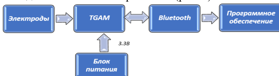
Рис.4. Структурная схема аппаратно-программного обеспечения одноканальной ЭЭГ
