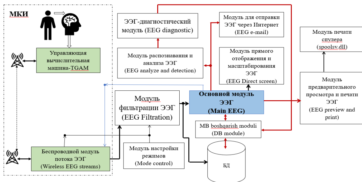
Рис.6. Структурная схема аппаратно-программного обеспечения для анализа ЭЭГ
