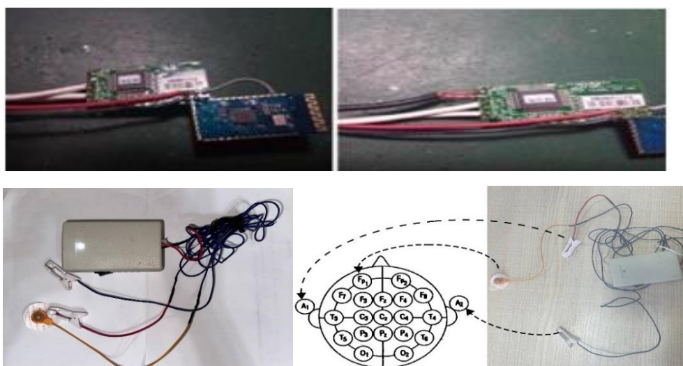
Рис.5. Одноэлектродный аппарат ЭЭГ и размещение электродов на головном мозге
