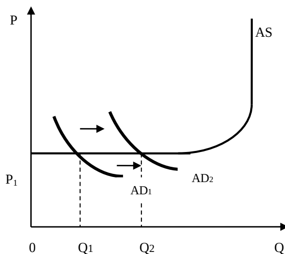
15.3-sızılma. Jatıq kósherde jalpı talap hám jalpı usınıs teńsalmaqlıǵınıń ózgeriwi
