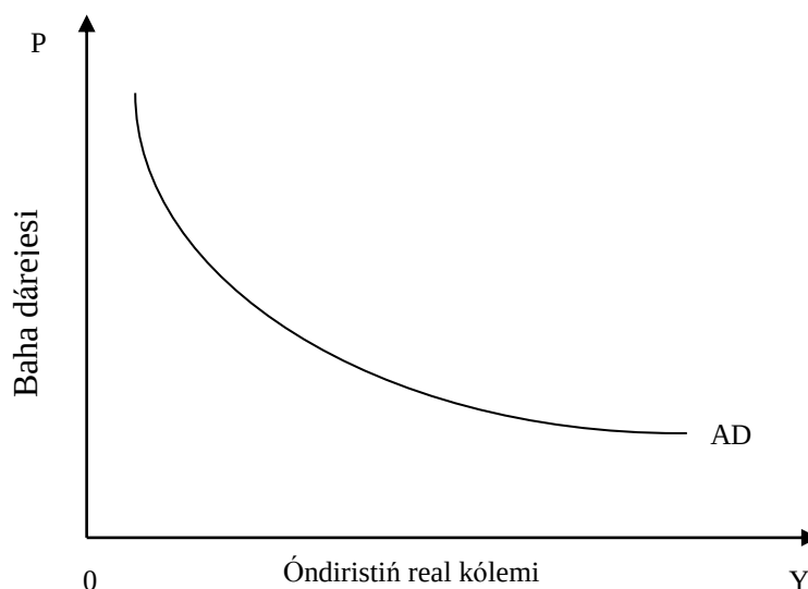
15.1-sızılma. Jalpı talaptıń qıya sızıǵı
