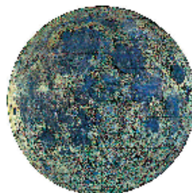
11-súwret. Aydiń kórinisi.
