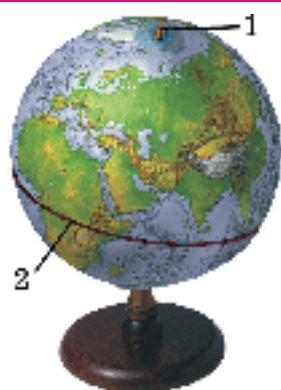
14-súwret. Globus: 1 – aylanıw kósheri; 2 – ekvator.
