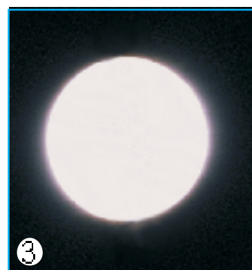
12-súwret. Aydıń ózgergen kórinisleri: 1 – jańa ay; 2 – yarım ay; 3 – tolıq ay.
