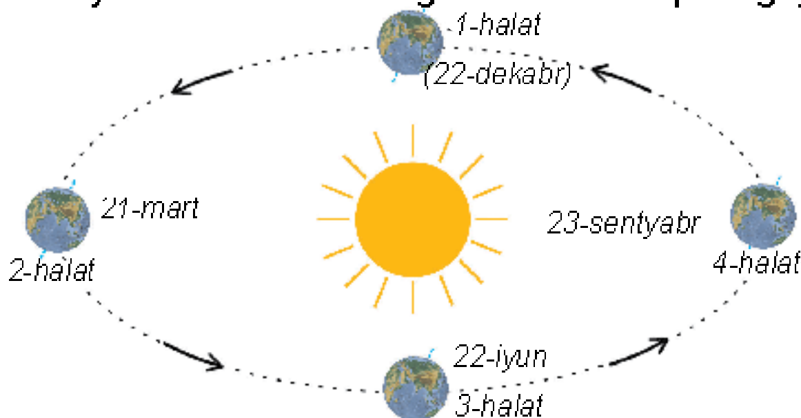
18-súwret. Jerdiń Quyash átirapında aylanıwı.
