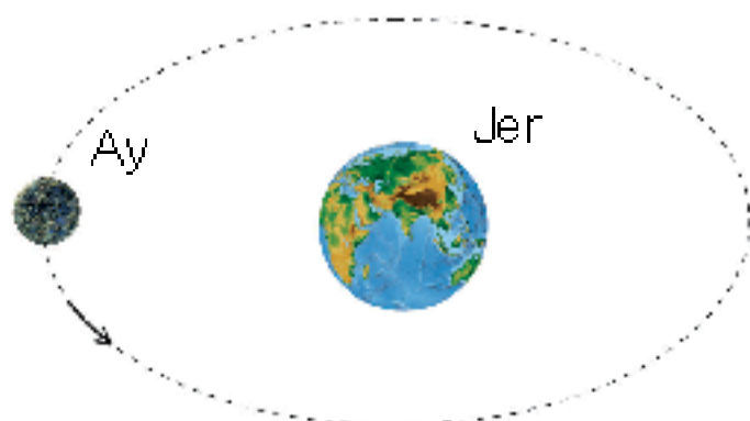
10-súwret. Aydiń Jer átirapında aylanıwı.
