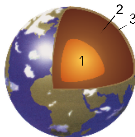
16-súwret. Jer sharınıń ishki dúzilisi.
