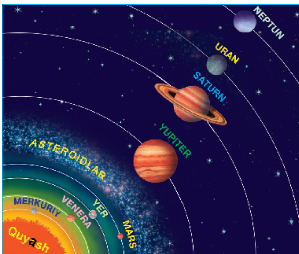
6-súwret. Quyash sistemasidaagi planetalar.
