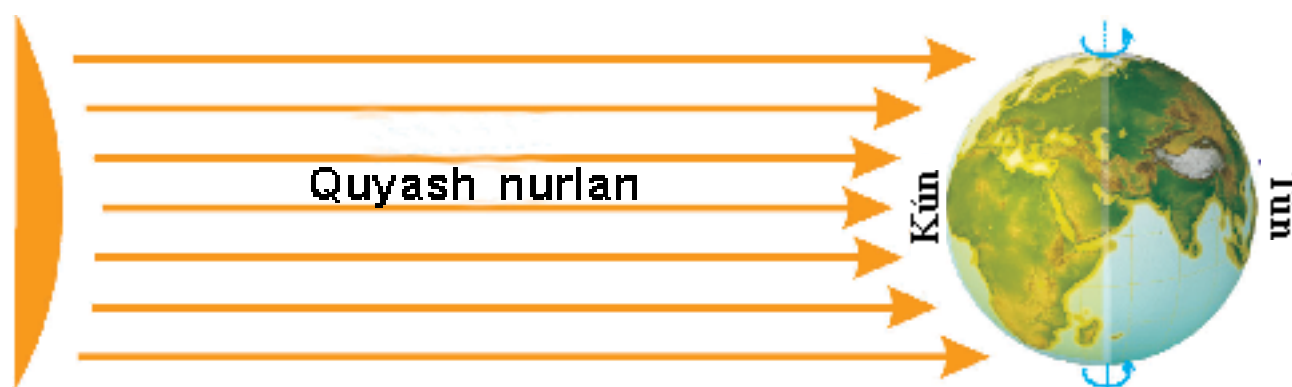
17-súwret. Kún hám túnniń almasıwı.
