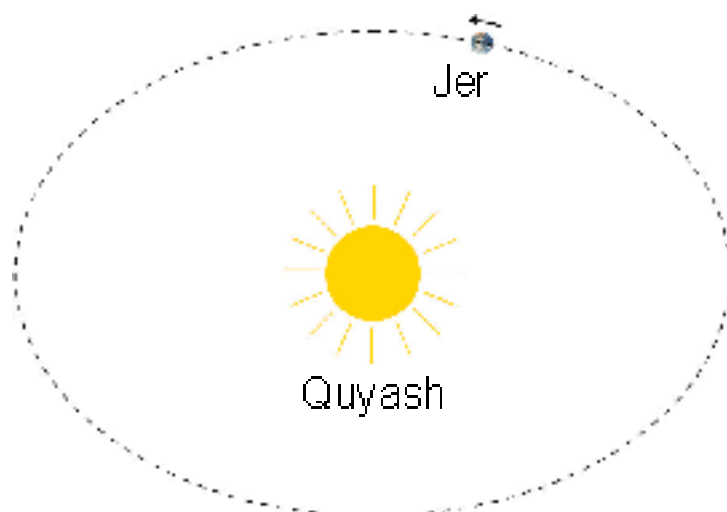
3-súwret. Jer Quyashtıń átirapında aylanadı.
