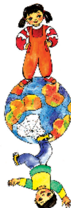
13-súwret. Jer ózine tartıp turadı.
