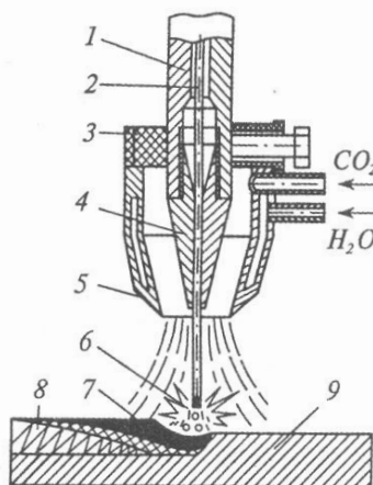
1-rasm. Karbonat angidrid gaz muhitida suyuqlantirib qoplama qoplash kallagining sxemasi:
