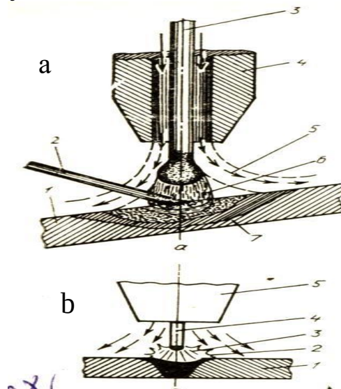
7.8-rasm. Argon muhitida suyuqlanmaydigan va suyuqlanadigan elektrodlar bilan elektr yoy yordamida payvandlash.
