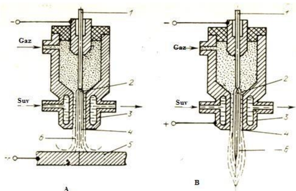
8.6-rasm. Plazma yordamida eritib purkash sxemasi.
