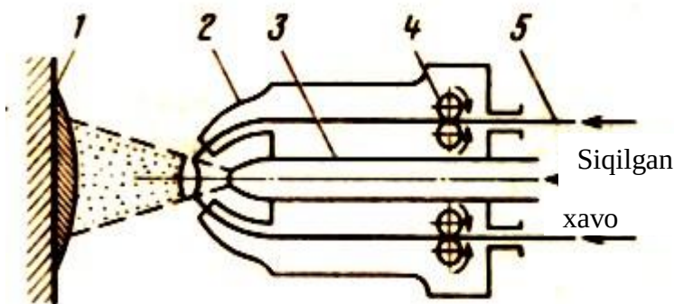
8.2-rasm. Elektr yoyi yordamida eritib qoplash jarayoni.
