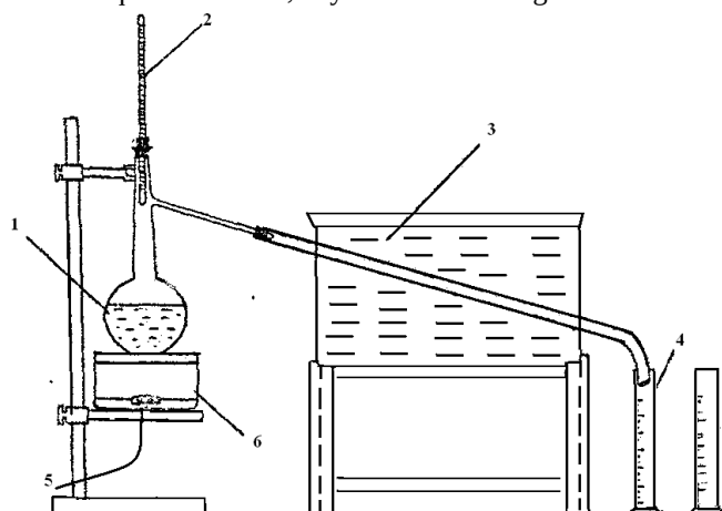
2-rasm. Benzinning fraksion tarkibini aniqlash asbobi.
