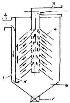
5.6-rasm. Statik se'erator: 1-kor'us; 2,3-kirituvchi va chiqa-ruvchi rezinali chig'anoq quvur-lar; 4-konussimon tarel-kalar; 5-qaytargichlar; 6-cho'kish minta-qasi; 7-cho'kindi to'kish jumragi.
