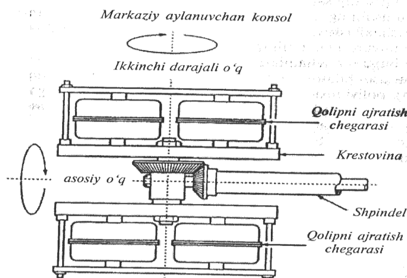
7- rasm. Ikki uqli rotatsion shakllash moslamasi.
