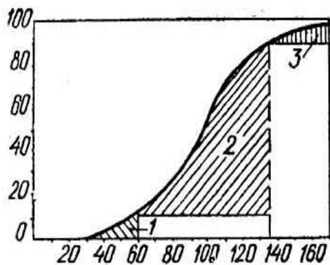
2.5-rasm. Benzinning fraksion tarkibi: 1-yurgizish fraksiyasi; 2-ishchi fraksiya; 3- og'ir fraksiya
