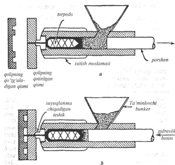
5-rasm. quyish mashinasining sxemasi: a-ochiq qolib, b-yo'iq qoli'.
