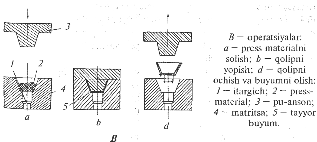
6-rasm. Com'ression 'resslash o'ratsiyalari sxemasi
