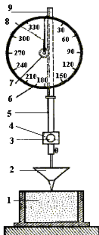
9-rasm. 'enetratsiya sonini aniqlash asbobi.
