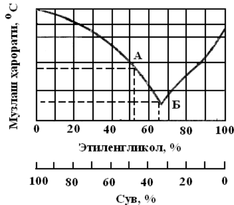
10-rasm ‘ast haroratda muzlaydigan etilin gilikolli suyuqlik larning muzlash haroratini etilenglikol tarkibiga boglash grafigi
