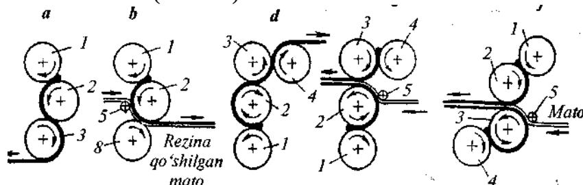
11-rasm. Rezina buyumlarni vulkanlash
