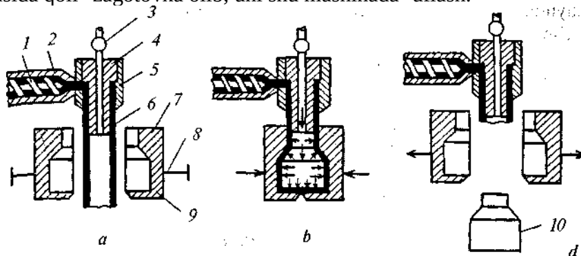
9-rasm. Ekstruziya usulida 'uflab ichi havol idishlar olish sxemasi: a - ekstruziya usuli bilan quvursimon zagotovka olish; b - zagotovkani 'uflash va buyum shakllash; d - buyumni olish. 1 - shnek; 2
