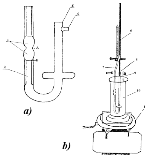
3-rasm. Ostvol d- 'inkevich viskozimetri.
