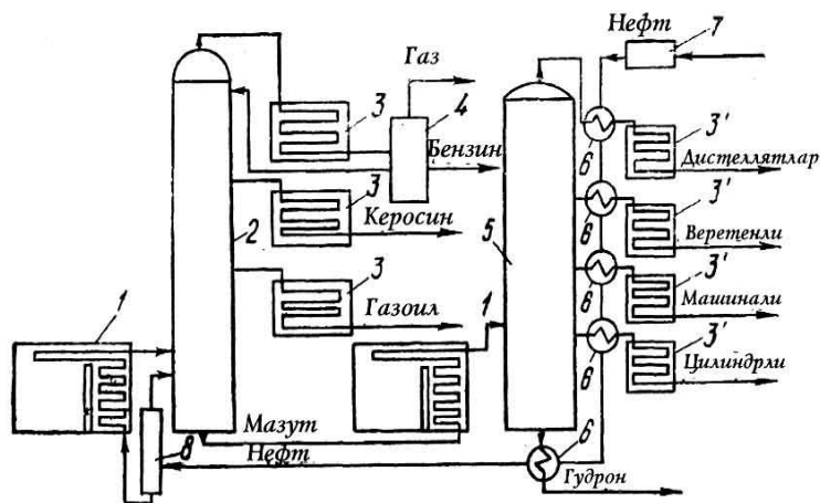
1.1-rasm. Neftni haydash qurilmasi: 1-quvurli ‘ech (isitgich); 2 va 5-rektifikatsion kolonnalar; 3-sovutgichlar; 4-kondensator-gaz ajratgich; 6-issqlik almashtirgich; 7-nasos; 8-bug‘lanish kolonnasi; quvurli vakuum isitgich.
