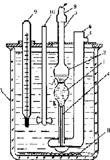
2.3-rasm. Kinematik qovushoqlikni aniqlash asbobi
