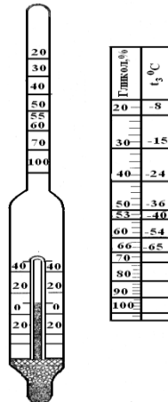
11-rasm Hidrometr va uning shkalasi
