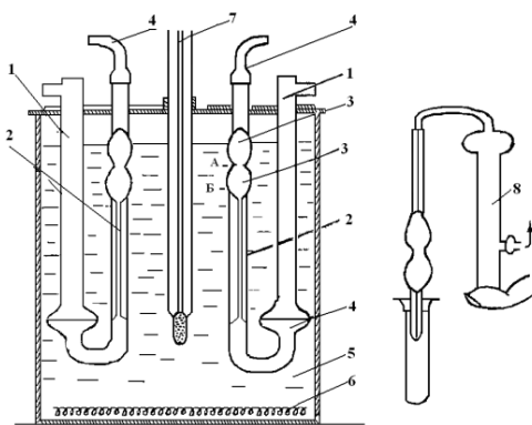
7-rasm. Suvli termostatga o'rnatilgan viskozimetрни umumiy ko'rinishi.
