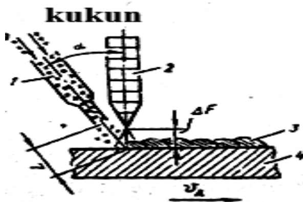
11.2-rasm. Kukunli eritib qoplash sxemasi: 1-eritib qoplanadigan kukun; 2- lazerli nurlanish; 3- eritib qoplangan valik; 4- ishlov beriladigan detalning sirti; V_d -ishlov beriladigan detalni siljitish tezligi; \alpha - kukunni kiritish burchagi; l - nurlanish fokusi bilan qoplanadigan sirt orasidagi masofa; L - kukun kiritilish oraliqi.
