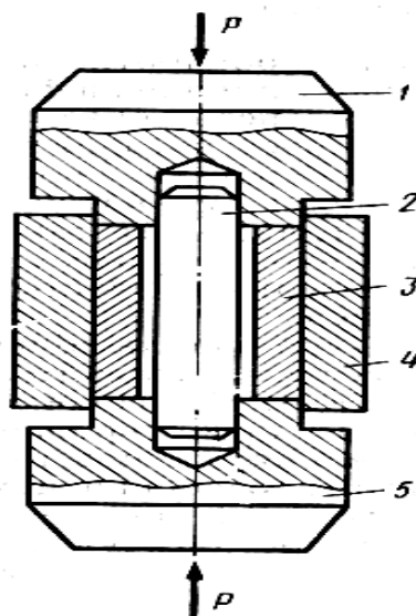
5.5-rasm. Detallarni cho'ktirish yo'li bilan tiklash.
