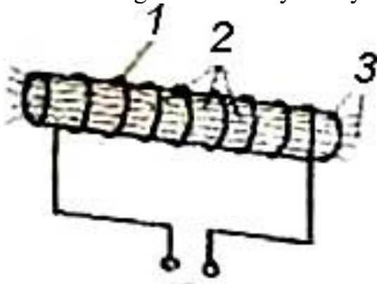
4.5-rasm. Tashqi yuzadagi ko'ndalang darzlarni aniqlashdagi bo'ylama usulda magnitlash sxemasi:
