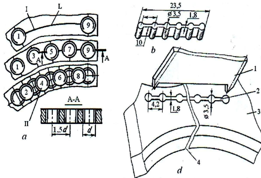
12.1-rasm. Yoriqlarni ta'mirlash
