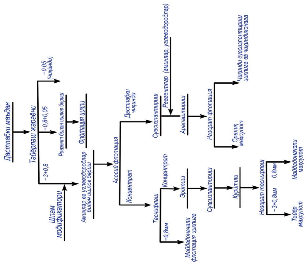
5.2 - расм. ФРАКЦИЯЛАРГА АЛОҲИДА ИШЛОВ БЕРИШ ВА ФЛОТАЦИЯЛАШ УСУЛИ БИЛАН ЙИРИК ЗАРРАЧАЛАРНИ ФЛОТАЦИЯЛАШ СХЕМАСИ
