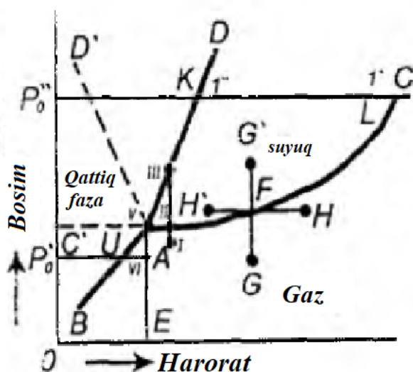
3.1-rasm. Oltingurgit tipidagi moddaning xolat diagrammasi
