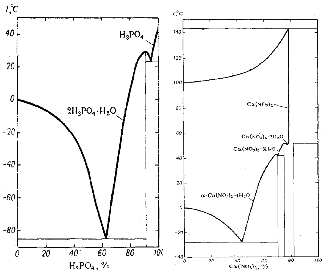
5.2-rasm. H_2O - H_3PO_4 ; H_2O - Ca(NO_3)_2 sistemaning holat diagrammasi.
