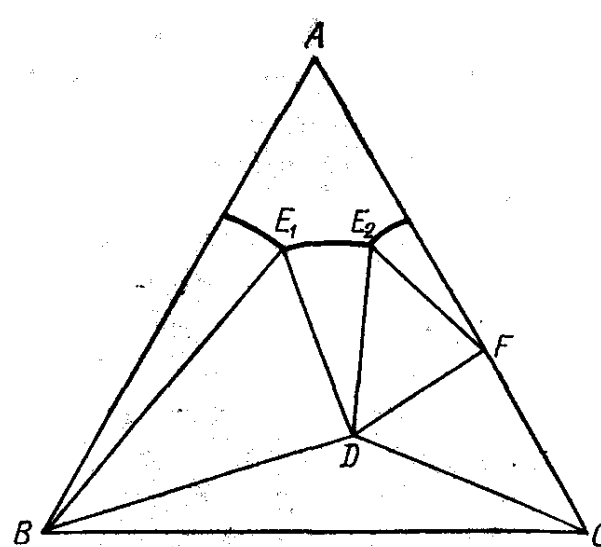
8.6-rasm. Suvli qo'shaloq tuz hosil qiluvchi uchlik sistema eruvchanlik izotermasi.
