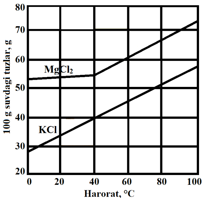
11.6-rasm. KCl va MgCl_2 ning turli haroratlardagi eruvchanligi.
