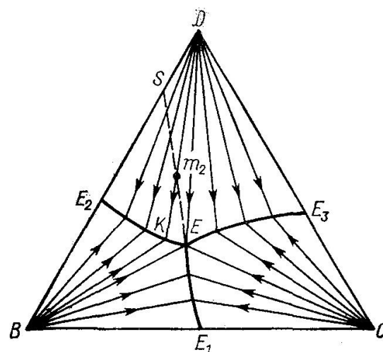
12.3-rasm. Xajmiy izotermiani markaziy aksi.
