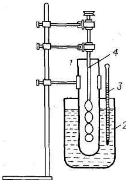
5.1-rasm Bir xil ionli to'rt komponentli sistemalar eruvchanligini izotermik usulda o'rganish. 1-probirka, 2-glitserinli hammom, 3-termometr, 4-aralashtirgich.
