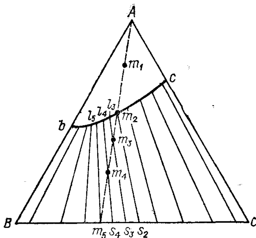
8.8-rasm. Aralash kristallarni uzliksiz qatorini hosil qiluvchi sistema izotermasi.
