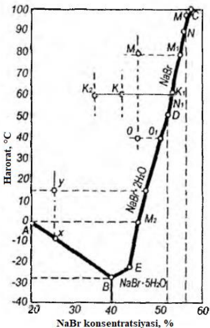
6.7-rasm. NaBr-H 2 O sistemasining eruvchanlik politermasi.
