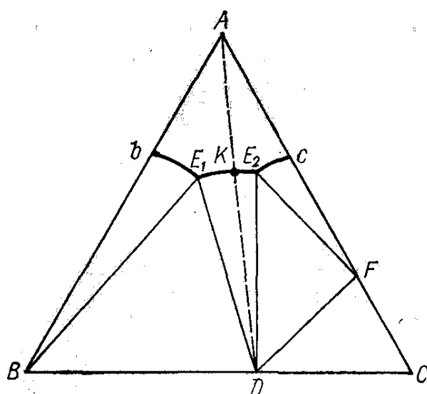
8.5-rasm. Suvsiz qo'shaloq tuz hosil bo'ladigan uchlik sistema eruvchanlik sistemasi.
