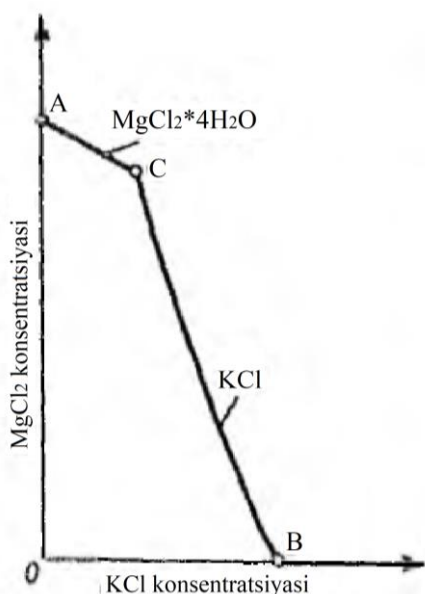
11.3-rasm. KCl-MgCl 2 -H 2 O sistemasining izotermasi (167,5°C dan yuqori haroratda).
