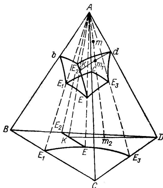
12.2-rasm. Xajmiy izotermiani markaziy aksini olish usuli.
