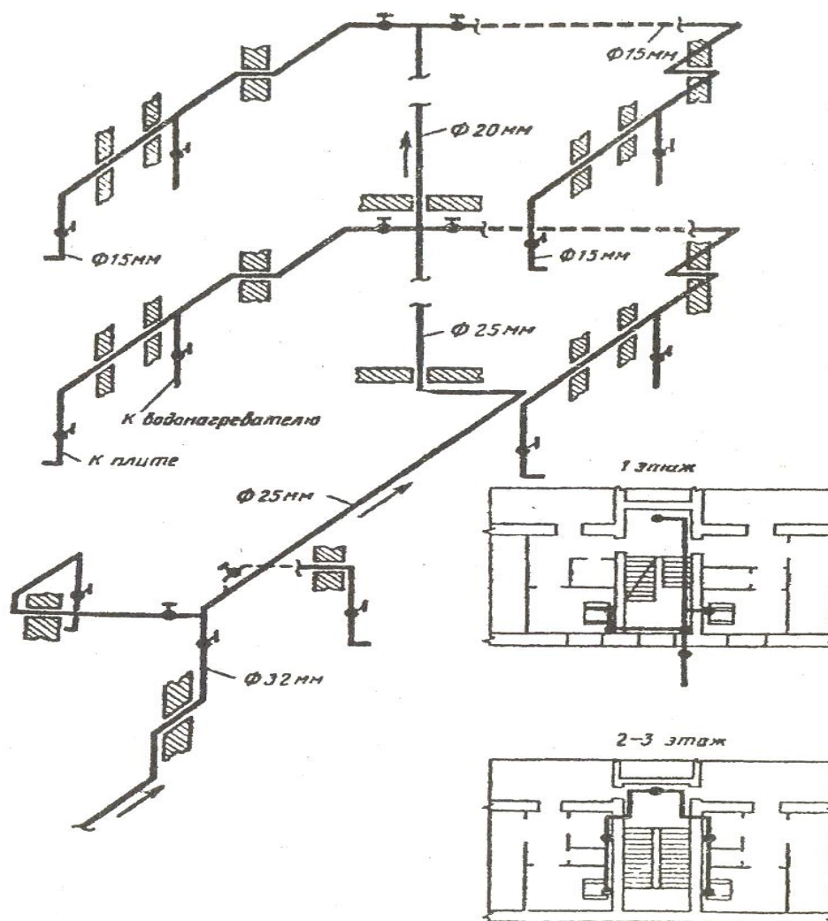
4.12-rasm. Turar-joy uy ichi gaz tarmog'ining sxemasi.
