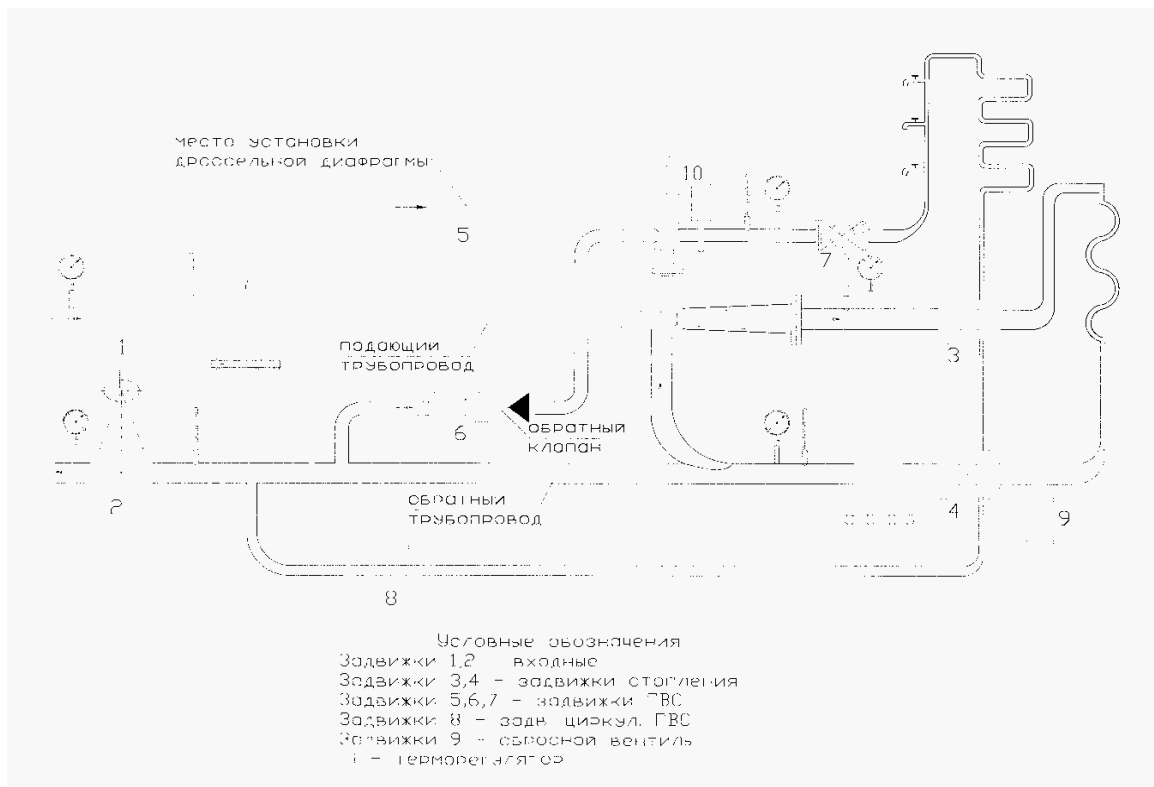
4.7-rasm. Issiqlik punktining sxemasi
