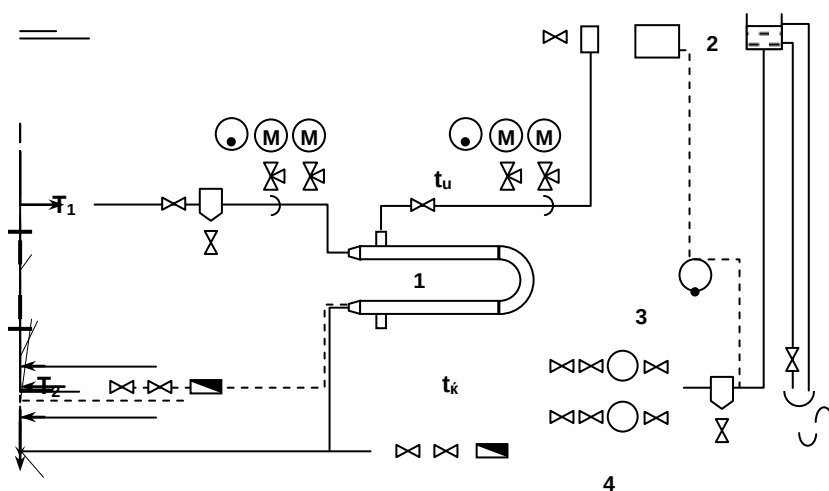
Yuqori haroratli issiqlik tashuvchi quvurlarga isitish tizimining «Bog‘liq bo‘lmagan holda» ulanish sxemasi.
