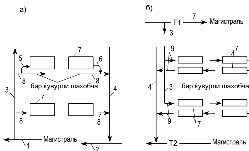
5.2-rasm Pastdan (a) va yo'qoridan (b) uzatuvchi suvli gorizontall isitish tizimlari: 1, 2 – uzatuvchi va qaytaruvchi magistral; 3 va 4 – uzatuvchi va qaytaruvchi tik quvur; 5 va 6 – uzatuvchi va qaytaruvchi ulama; 7 – isitish asboblari; 8 – bir quvurli shaxobcha; 9 – bifilyar tarmoq.
