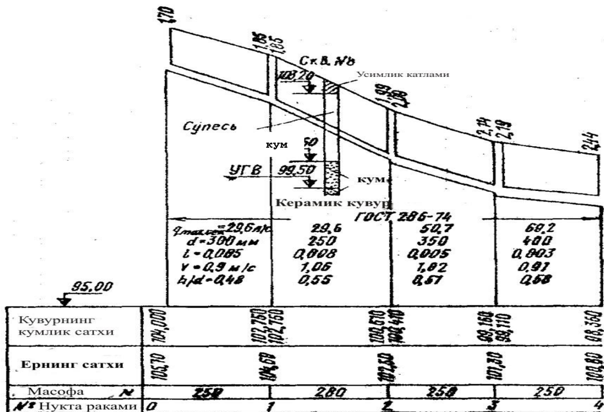
3-sxema. Kanalizatsiya tarmog'i profili.
