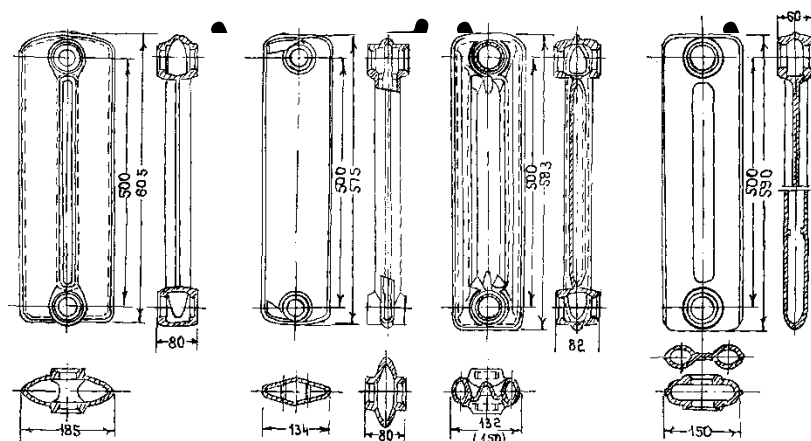
4.3-rasm. Turli isitish asboblarining shakli: a – «Polza» radiatori; b – «Gigiyenicheskiy» radiatori; v – «Moskva-132» radiatori; g – LOR-150 nomli radiator.
