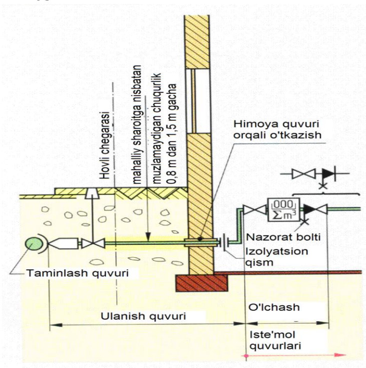
Ichimlik suvi quvurini turar joy binosiga o‘rnatish sxemasi.
