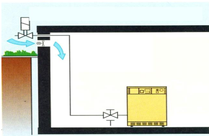
Ventiliyatorli shamollatish tizimi. Gaz-magnit ventili ventiliyator o'chib qolgan holda gazni yopadi.
