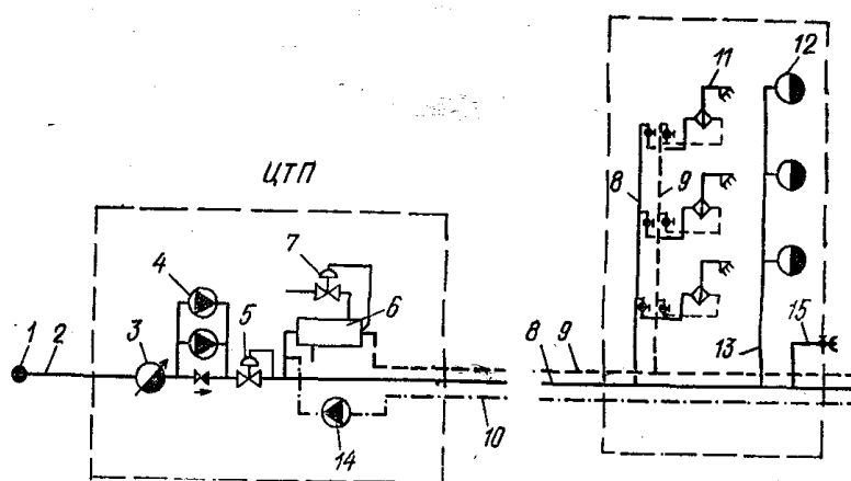
Rasm 1.4. Shohsimon suv ta'minoti tarmoqlarining sxemasi
