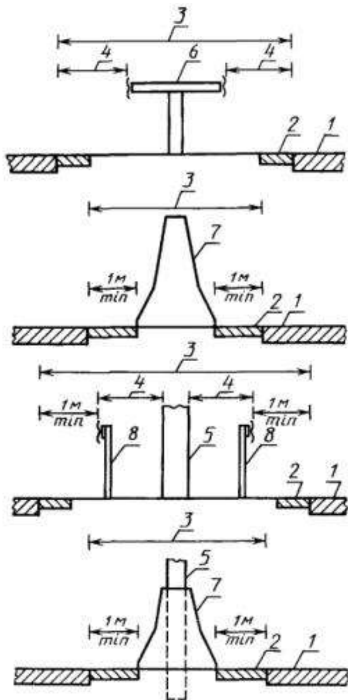
1 qatnov qismi; 2 - kraevaya ukrepitelnaya polosа; 3 - shirina razdelitel'noy polosы; 4 - raschetnyy poperechnyy progib ograjdeniya; 5 - prepyatstvie; 6 - baryernoe dvustoronnee metallicheskoе ograjdenie; 7 - dvustoronnee jelezobetonnoe ograjdenie parapetnogo tipа; 8 - baryernoe odnostoronnee metallicheskoе ograjdenie
