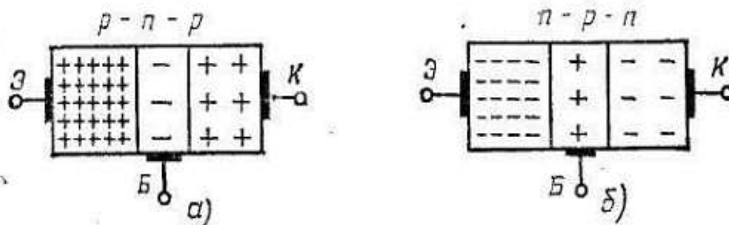
2-расм. p-n-p (а) ва n-p-n (б) типли биоляр транзисторларнинг структураси
