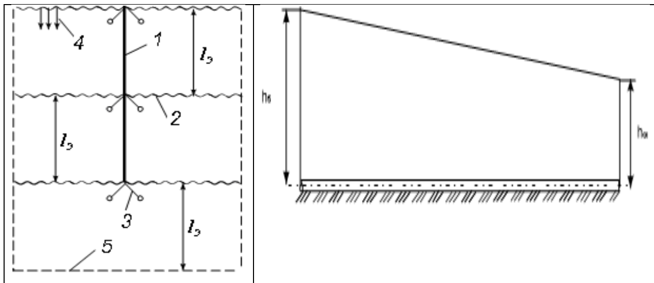
2.8.1-чизма. Кўчма суғориш қувурлари ёрдамида суғориш: 1—шоҳ ариқ (нов); 2—кўчма суғориш қувури; 3—сув чиқариш мосламаси; 4—суғориш эгати; 5—суғориш даласи чегараси
