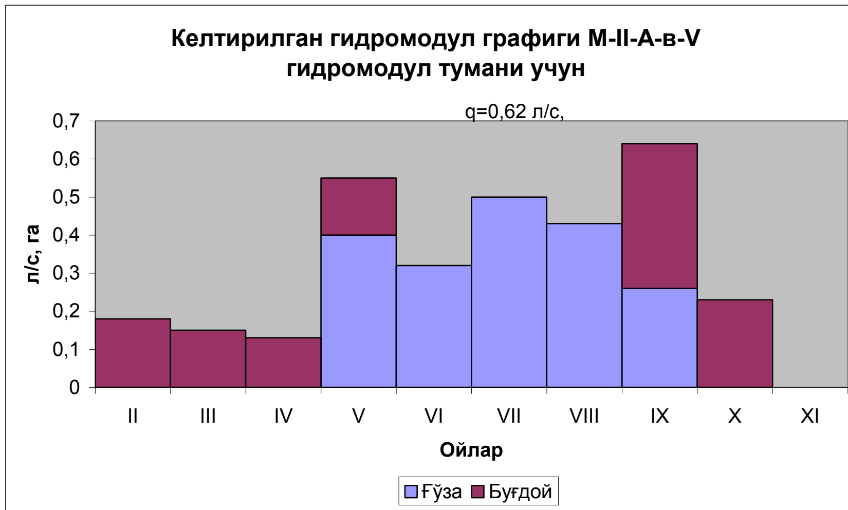
2.4.1-чизма. “Салоҳиддин бобо Савриддин ” фермер хўжалигининг келтирилган гидромул графиги
