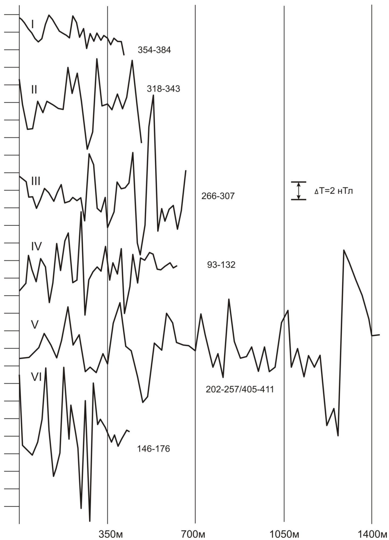
Рис.14. Изменение магнитного поля по профилям I-VI микромагнитной съемки (площадь железорудной конкреции).
