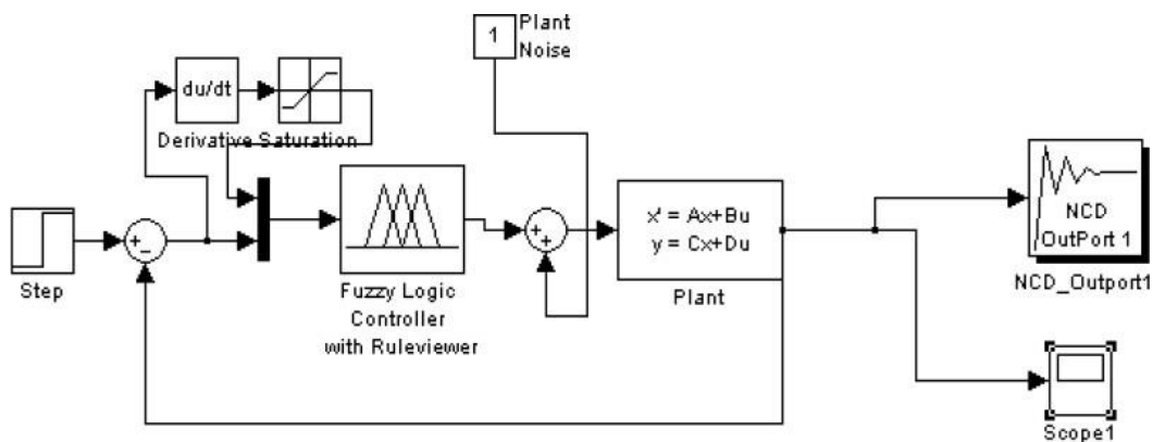
4-расм. Ноаниқ ростлагичли (Fuzzy Logic Controller) автоматик ростлаш тизимининг структуралӣ схемаси
