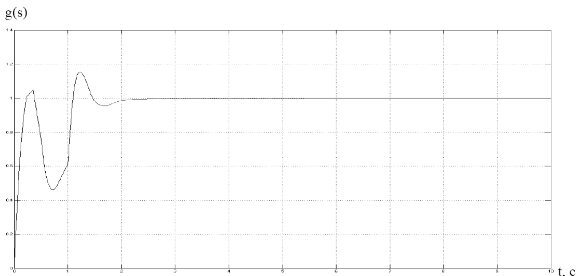
5-расм. Топширик канали бўйича ноаниқ автоматик ростлаш тизимининг ўткинчи жараёни 7 ва 8-расмлардан кўриб турганингиздек, яъни ҳар иккала ростлаш тизими ҳам объект
