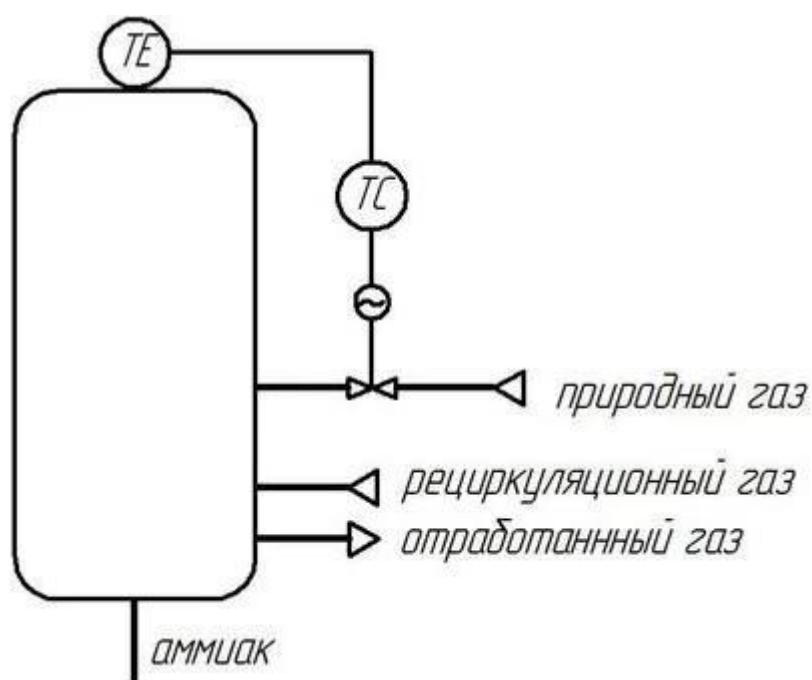
Рисунок 2. Сокращенная функциональная схема объекта управления
