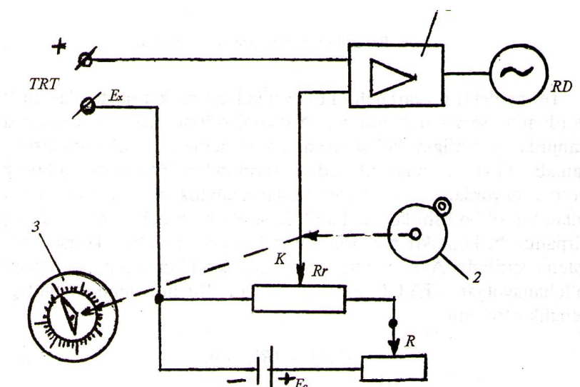
36- rasm. Elektron avtomatik potensiometrning sxemasi.
