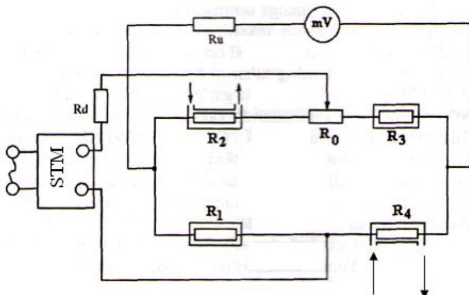
81- rasm. Termokonduktometrik gaz analizatorining printsiplial o'lchash ko'priki sxemasi.
