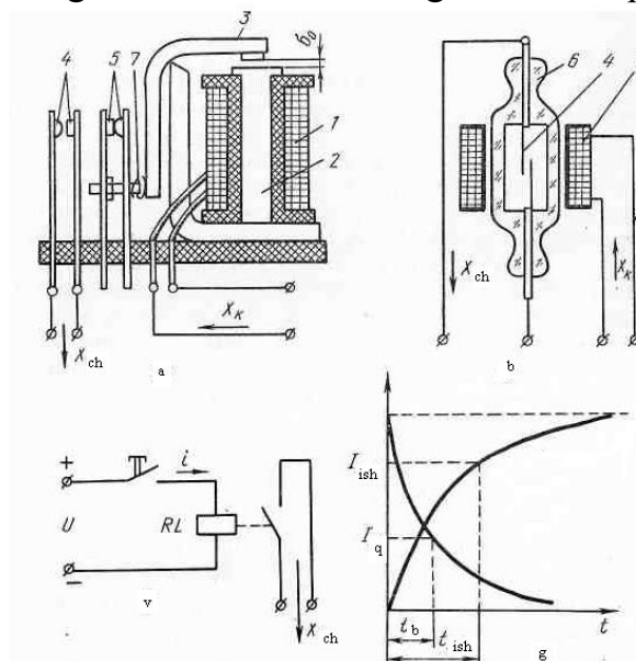
83- rasm. O'zgarimas tok relesi: a-aylanuvchi yakorli rele; b-yakorsiz rele (gerkon); v-releining elektr sxemasi; g - releining dinamik tavsif grafiklari; 1 -elektromagnit g'altagi (o'ramasi), 2 – qo'zg'almas po'lat o'zak; 3-o'zak (yakor), 4 - toksiz holatdagi ochiq kontakt, 5 - toksiz holatdagi yopiq kontakt, 6-shisha kolbacha.
