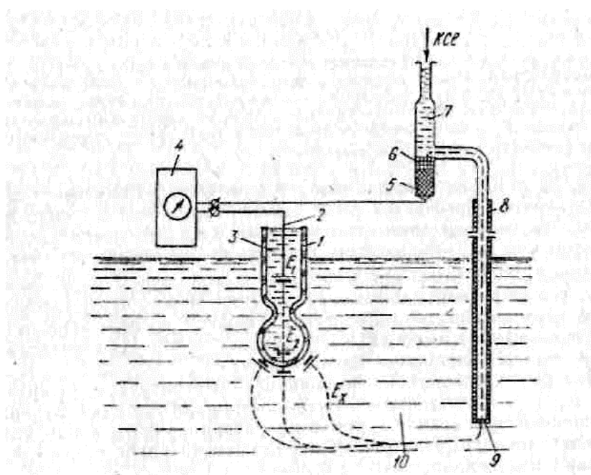
73- rasm. Shisha va elektrolari bo'lgan pH – metr
