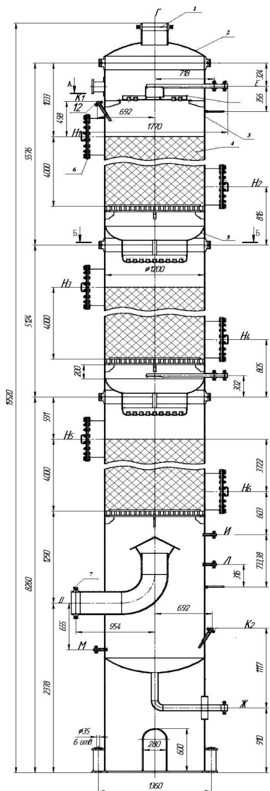
3-расм. Насадкали абсорбер:
