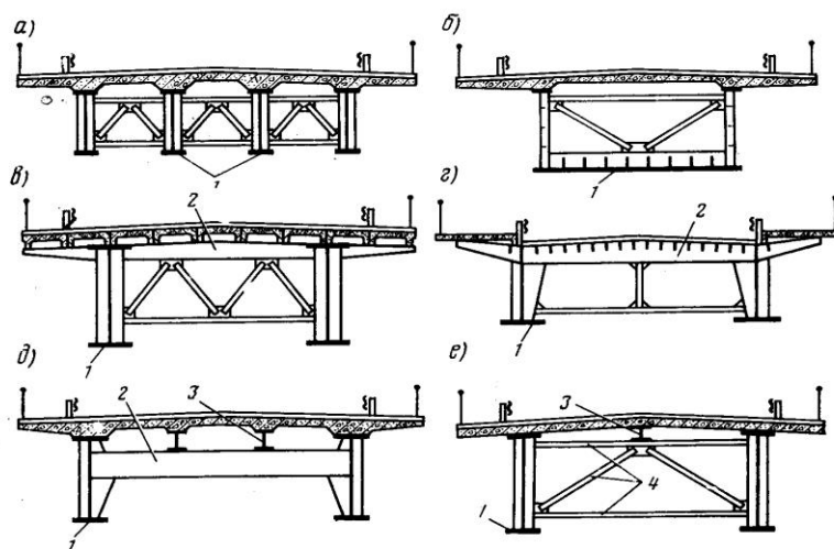
Рис. 22.4. Конструкция балочной клетки: 1 — главная балка; 2 — поперечная балка; 3 — продольная балка; 4 — поперечная балка, объединенная с поперечными связями пролетного строения
