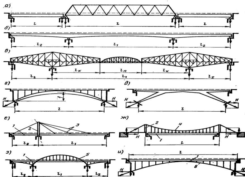
Рис. 21.7. Основные системы металлических мостов: 1 — балка жесткости; 2 — пилон; 3 — вант; 4 — кабель; 5 — арочный пояс; 6 — подпружиненная гибкая арка
