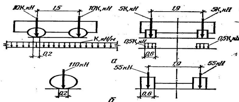
Рис. 1.1. Схема временной нормативной вертикальной нагрузки АК (размеры в м): а — полосовая нагрузка и двухосная тележка; б — одноосная тележка
