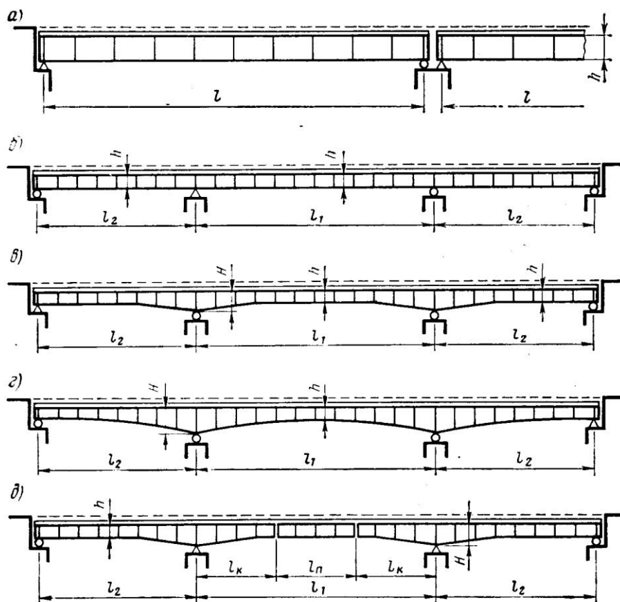
Рис. 22.1. Системы мостов со сплошными балками
