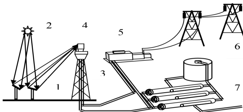
2.1.1-rasm. Minorasimon quyosh elektr stantsiyasining printsipl sxemasi
