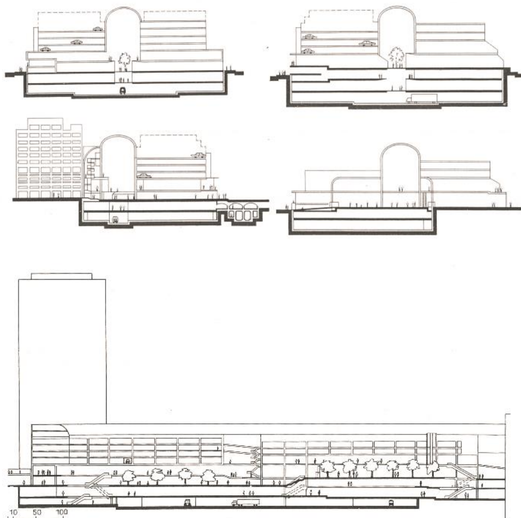
Рис. 6.4. Пешеходная зона Центра им. Итона в Торонто. Продольный разрез
