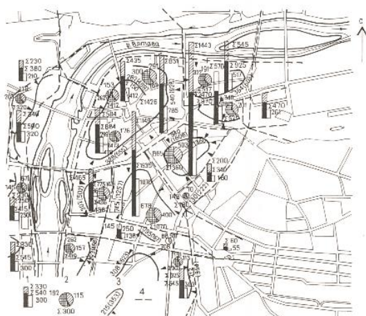
Рис. 7.14. Потребности в автостоянках и возможности развития их сети в центре Праги 1 — общая потребность; 2 — потребность для населения; 3 — потребность для служебного транспорта; 4 — границы зон.
