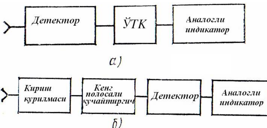
8.5–расм. ўзгарувчан кучланиш анологли электрон вольтметрнинг структура схемаси.
