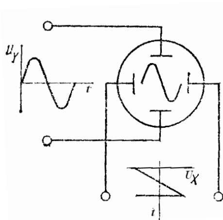
8.2 – расм. Разверткание вѣт
