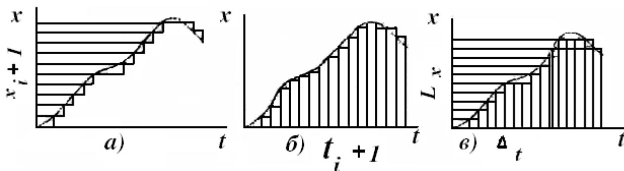
8.7– рasm. Сигналларни квантлаш йўли билан дискрет кўринишга айлантириш
