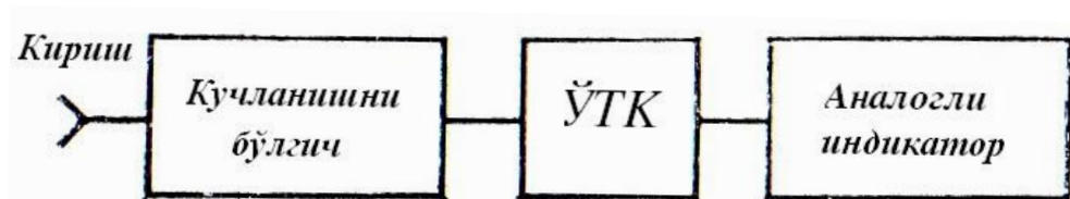
8.4– расм. Аналогли электрон вольтметр структура
