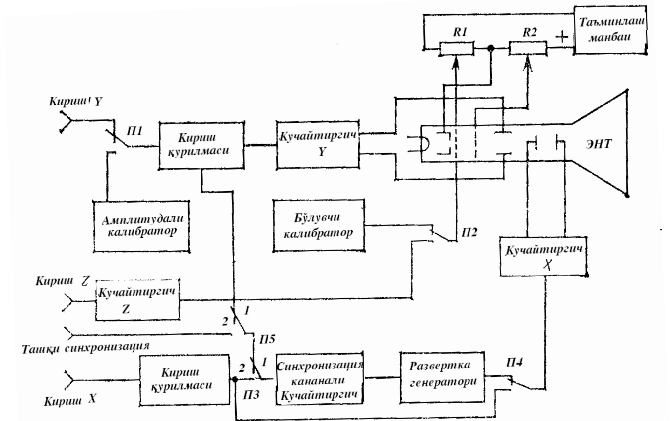
8.1–расм. Электрон нур осциллографининг структура схемаси
