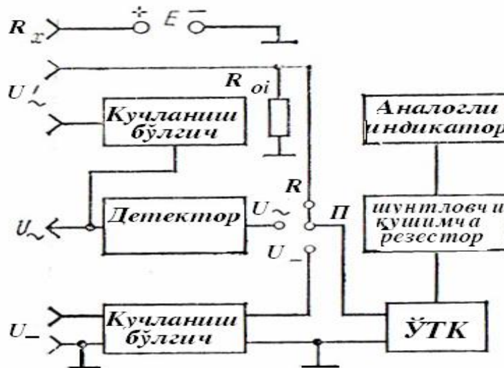
8.6–расм. Универсал аналогли электрон вольтметрнинг структура схемаси.
