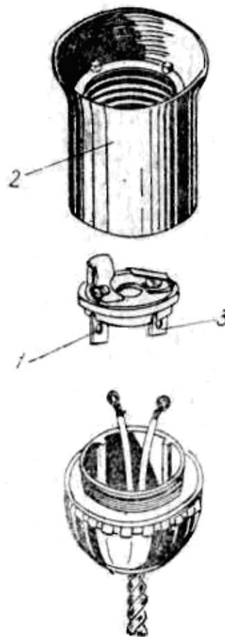
2-расм. Патронни йиғиш: 1,3 – контактлар, 2 – корпус
