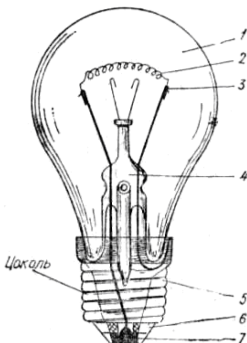
1-расм. Електр лампа ва унинг тузилиши
