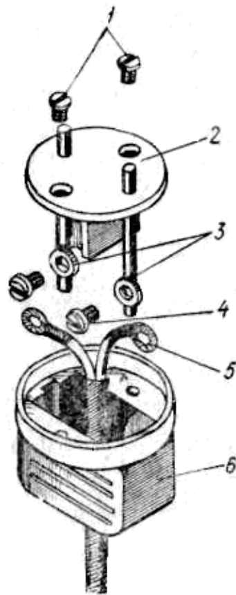
1-расм. Електр вилкасининг тузилиши
