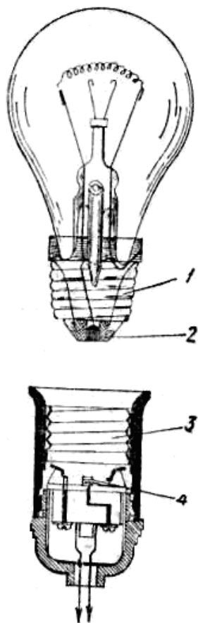
3-расм. Електр патрон лампаси билан: 1-винт, 2-контакт, 3-ички винт, 4- контакт
