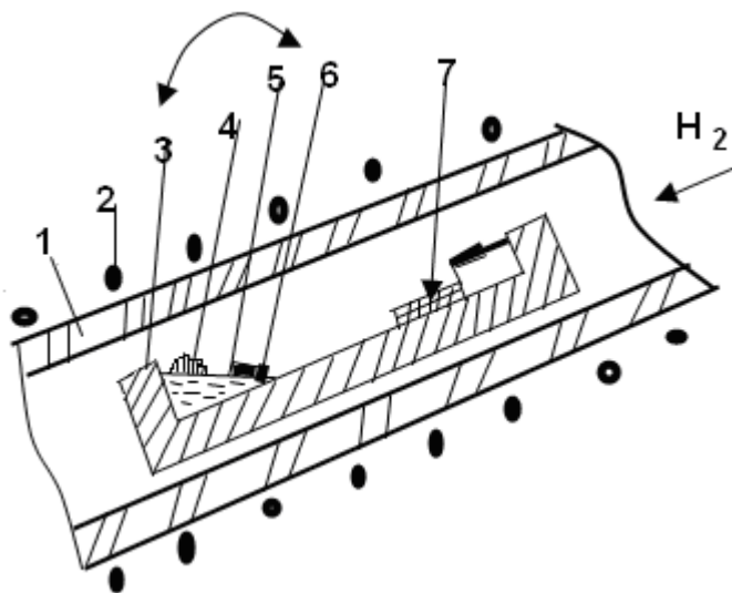
5-расм. Нелсон усули бўйича суюқ эпитаксия учун контейнер схемаси: 1-Кварс реактор; 2-қаршилик электр печи; 3-графит қайиқча; 4-модда-манба; 5-лигатура; 6-эритма (гелий); 7-таглик.
