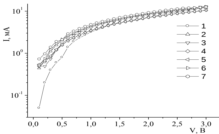
9-расм. pSi-n(Si_2)_{1-x}(CdS)_x ( 0 \leq x \leq 0.01 ) тузилманинг BAX, тўғри чизиqli қисмининг яримлогорифмик ўлчамида турли хароратлар учун графиклари ўлчанган қийматларига эга эканлигини кўриш мумкин. Бундай боғланиш учун р-п тузилмалар учун В.С.Стафив томонидан қуйидаги муносабат аниқланди.
