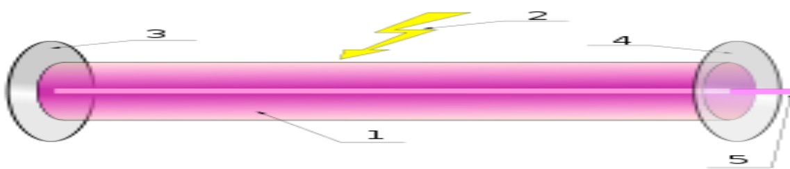
3.7- Rasm. Geliy – neonli lazerning kvartslı gaz razryadli trubkasining umumiy ko'rinishi: 1- ishchi muhit, 2- lazer nurini hosil qiluvchi energiya, 3- tınıqmas kuzgu, 4- yarım tınıq kuzgu, 5-lazer nuri
