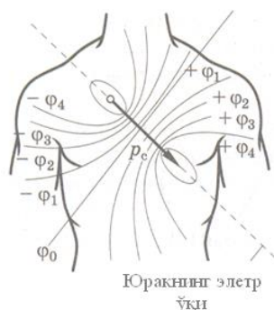
2.10 - Rasm. Yurak dipol momenti R_{yu} vektorining vaziyati va dipolmomenti maksimal bo'lgandagi vaqt momenti uchun ekvipotentsial chiziqlarning hosil bo'lishi
