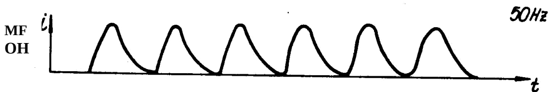
3.15- Rasm. Biryarimdavrli uzluksiz (OH) - 50 Gts chastotali eksponentsial qirqimli sinusoidal formadagi tok impulslari
