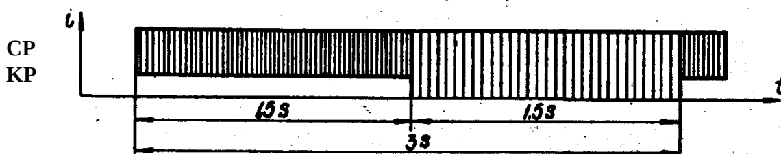
3.18 -Rasm. Qiska davr (KP) - OH ko'rinishidagi tok impulslari seriyasining DH ko'rinishli tok impulslari seriyasi bilan almashinishi
