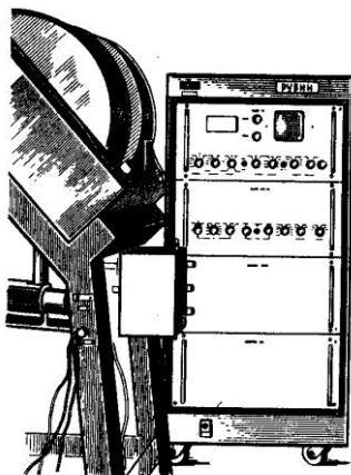
2.50 – Rasm. «Rubin» EPR spektrometrining umumiy ko'rinishi
