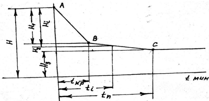
8-расм. Қуюлтириш эгри чизиғи
