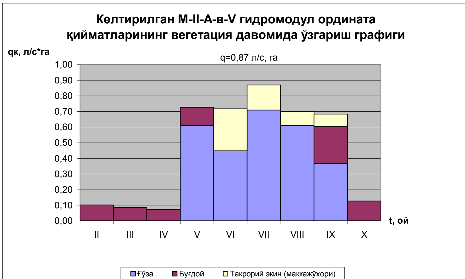
3.3.1-чизма “Бўстонназар” фермер хўжалигининг келтирилган гидромодул графиги
