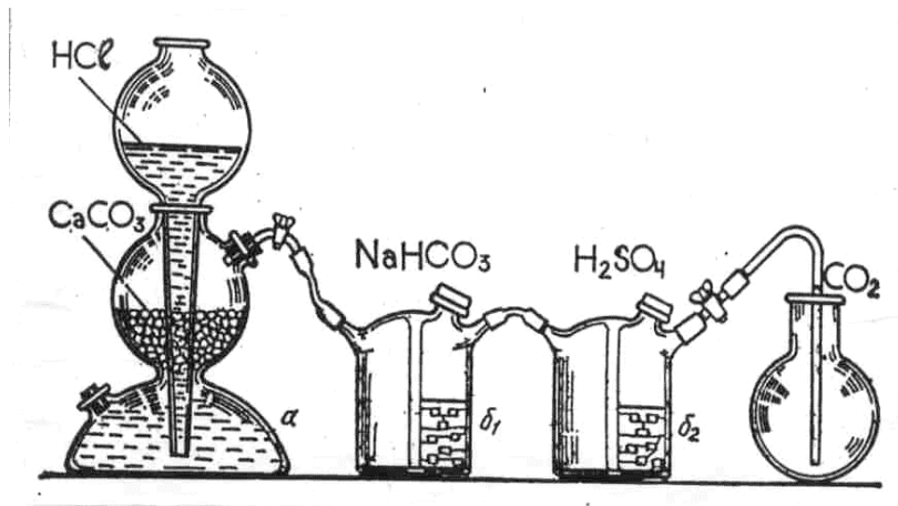
9-rasm. Karbonat angidrid olinadigan qurilma:
