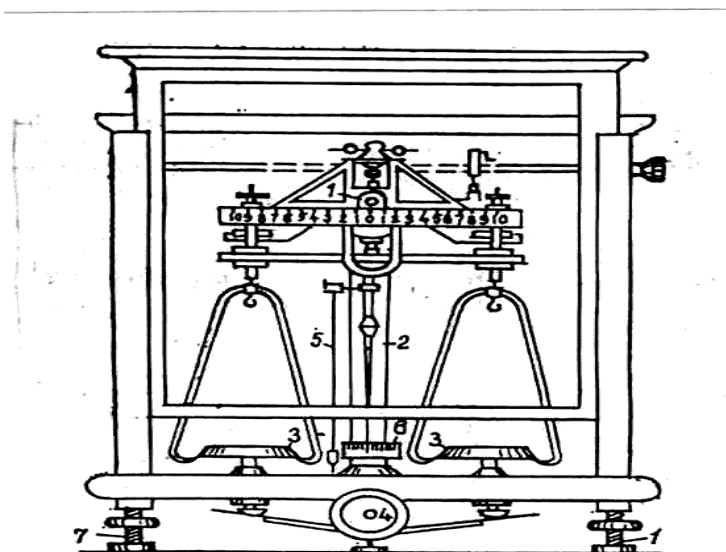
2-rasm. Analitik tarozi:
