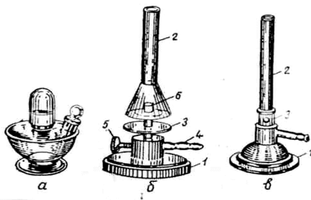
3-rasm. Spirt lampasi va gaz yondirgichlari:
