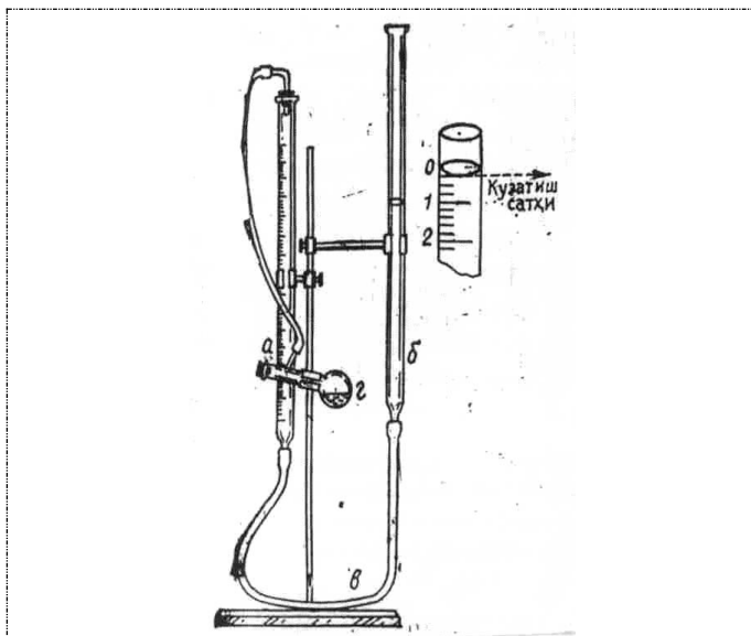
10-rasm. Vodorodni siqib chiqarish usuli bilan metall ekvivalentini aniqlovchi asbob:
