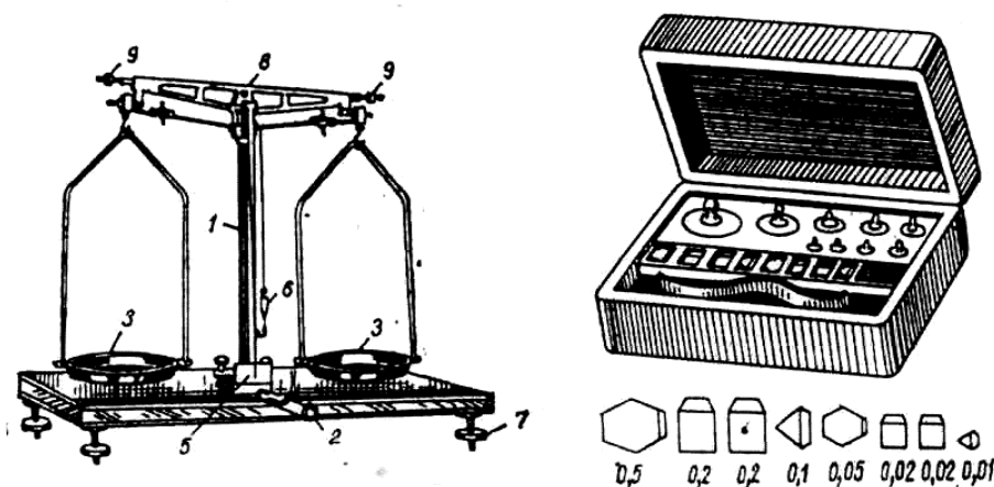
1-rasm. Texnokimyoviy tarozi va uning toshlari:
