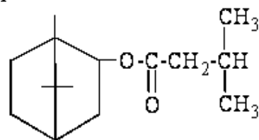
Bornilizovalerianat
