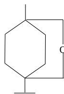
Sineol
