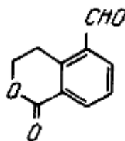
eritrotsentaurin
