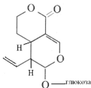
sverozid
