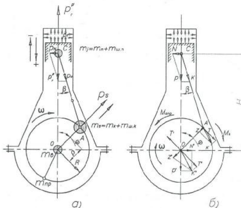
6-rasm. Markaziy krivoship - shatun mexanizmiga ta'sir etuvchi kuch va momentlar:
