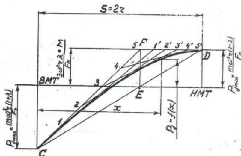
9-rasm. KShM ning ilgarilanma-qaytma qismlari inersiya kuchlarining diagrammasi
