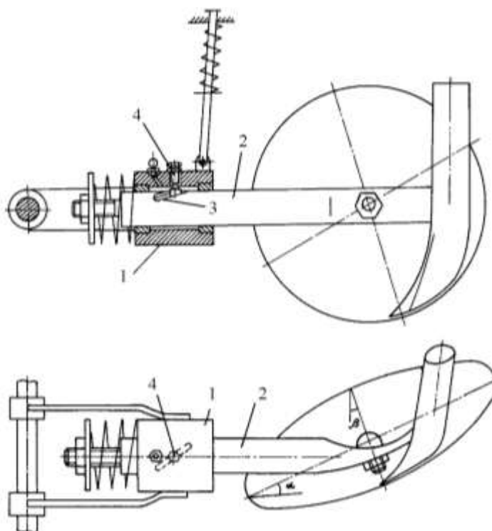
1.6-рasm. Битта дискли сошник
