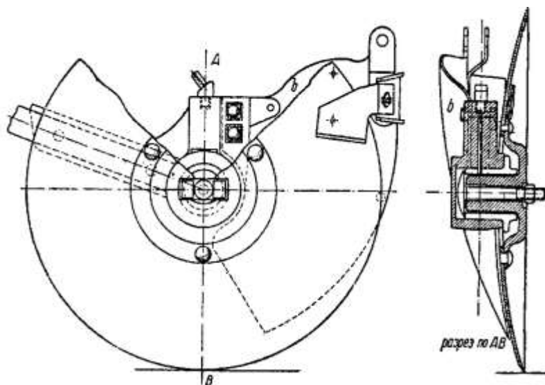
1.5-рasm. Битта дискли сошник
