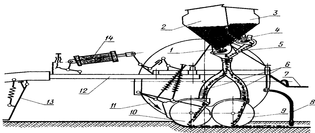
1.1-расм СЗТ-3,6 экиш машинасининг технологик схемаси
