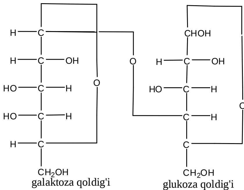
laktoza
