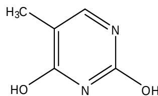
timin (2,6 -digidroksi - 5 -metilpirimidin)
