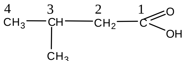
3 -metilbutanat kislota
