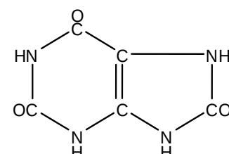
siydik kislotasi
