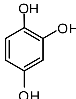
1,2,4 -benzotriol gidroksogidroxinon 1,2,4 - trigidroksibenzol
