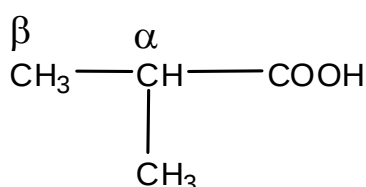
\alpha -metilpropion kislota
