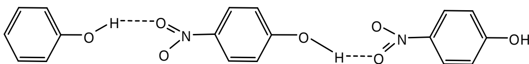
Molekulalararo asosilangan p -nitrofenol
