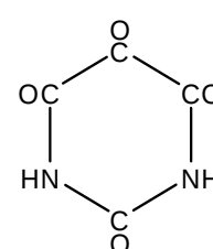
allksan
