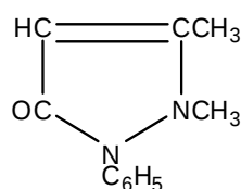
antipiridin
