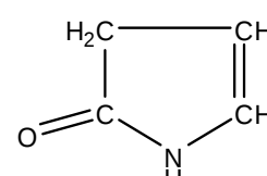
pirazolon
