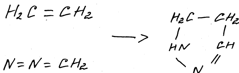
Pirazolin
