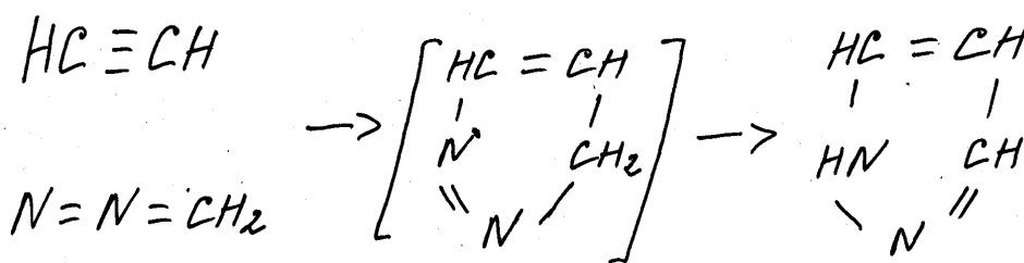
Pirazol
