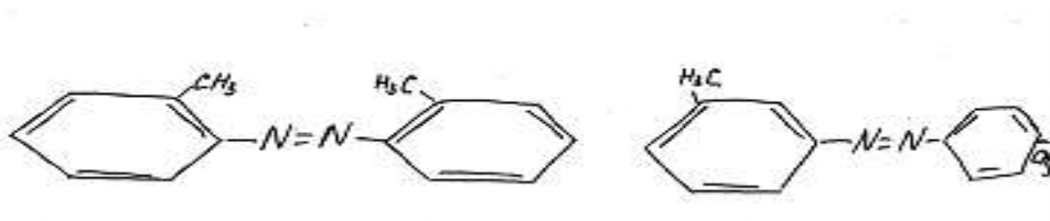
O_1O^1 -Azotoluol
