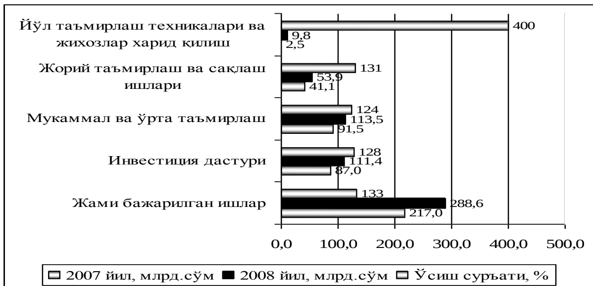
2.2-расм. Умумий фойдаланишдаги автомобиль йўлларида қуриш ва таъмирлаш кўрсаткичлари
