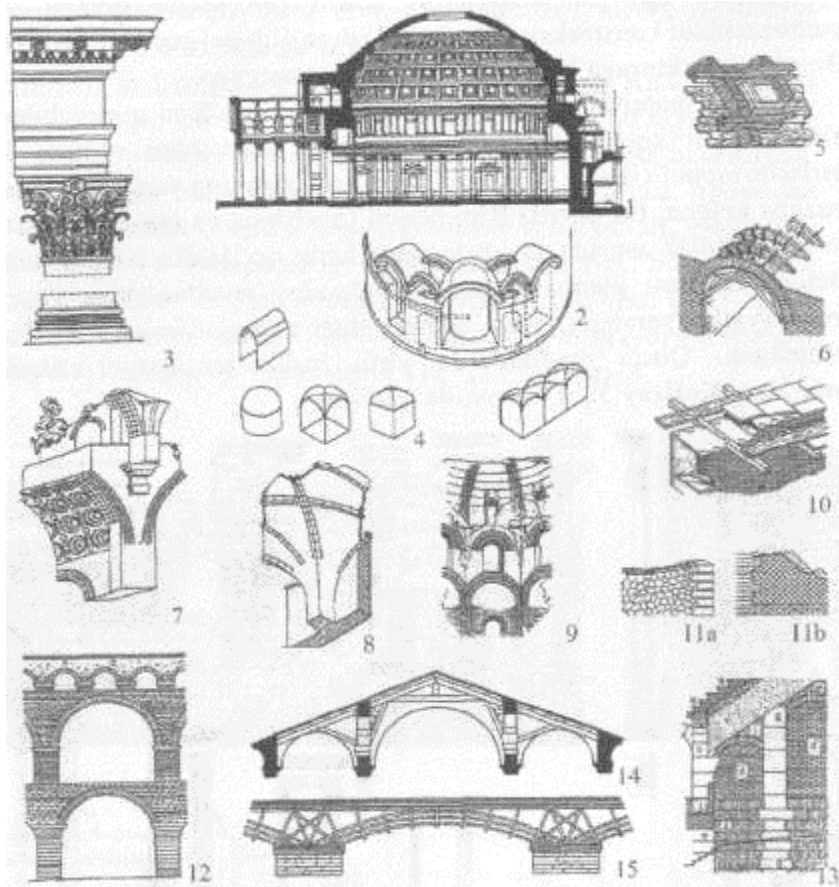
Qadimgi Rim arxitekturasida konstruksiyalar.
