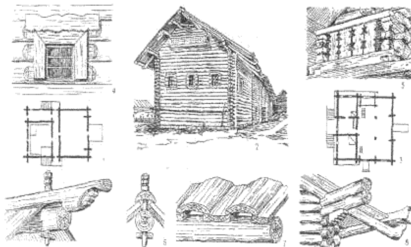
Qadimgi rus turar -joy binolari va ularning konstruktiv detallari.
