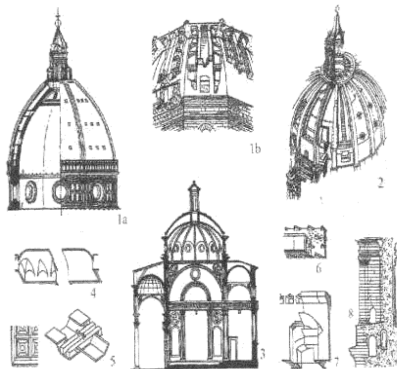
Uyg'onish davri arxitekturasining konstruksiyalari va qurilish usullari.
