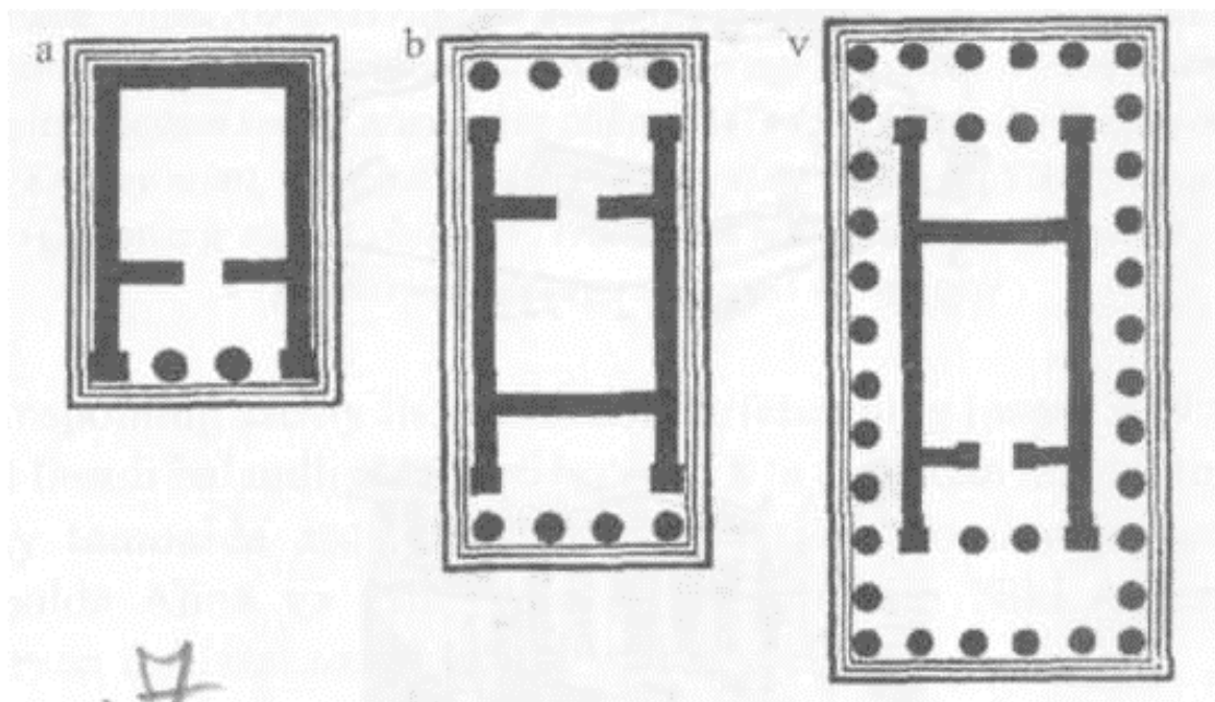
Qadimgi Yunon ibodatxonalarining tiplari.
