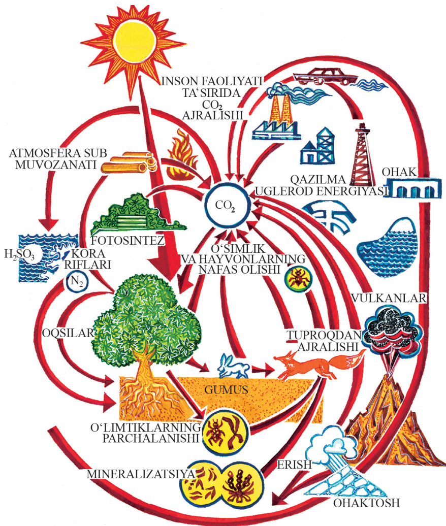
76-rasm. Biosferada uglerodning davriy aylanishi.
